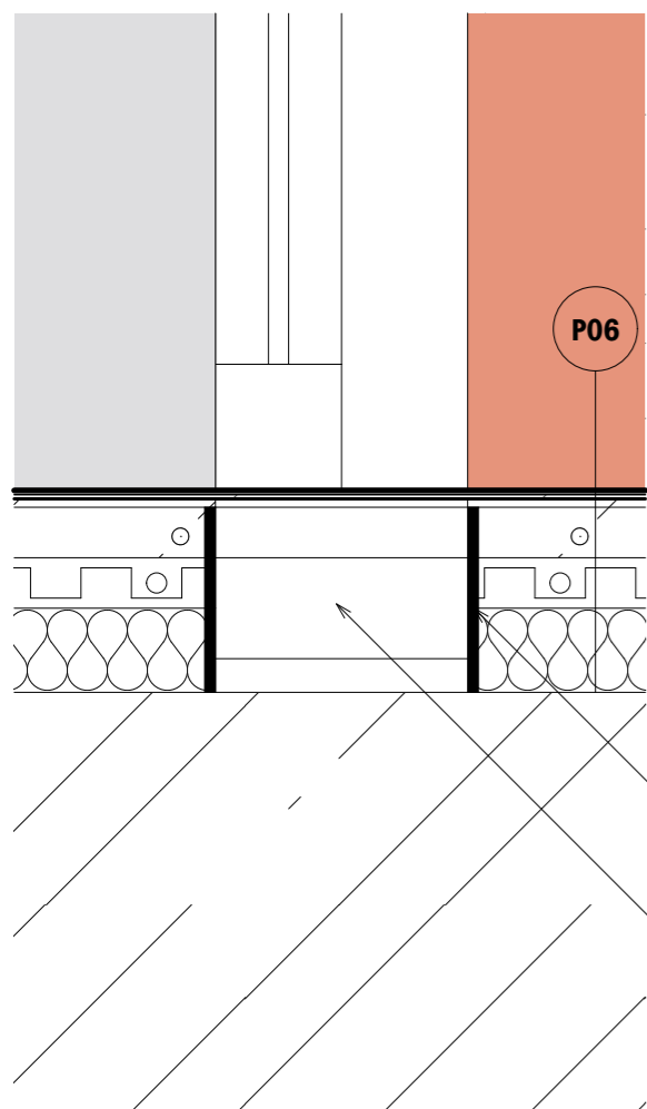
Detail parapetu posuvných dverí M 1:5
