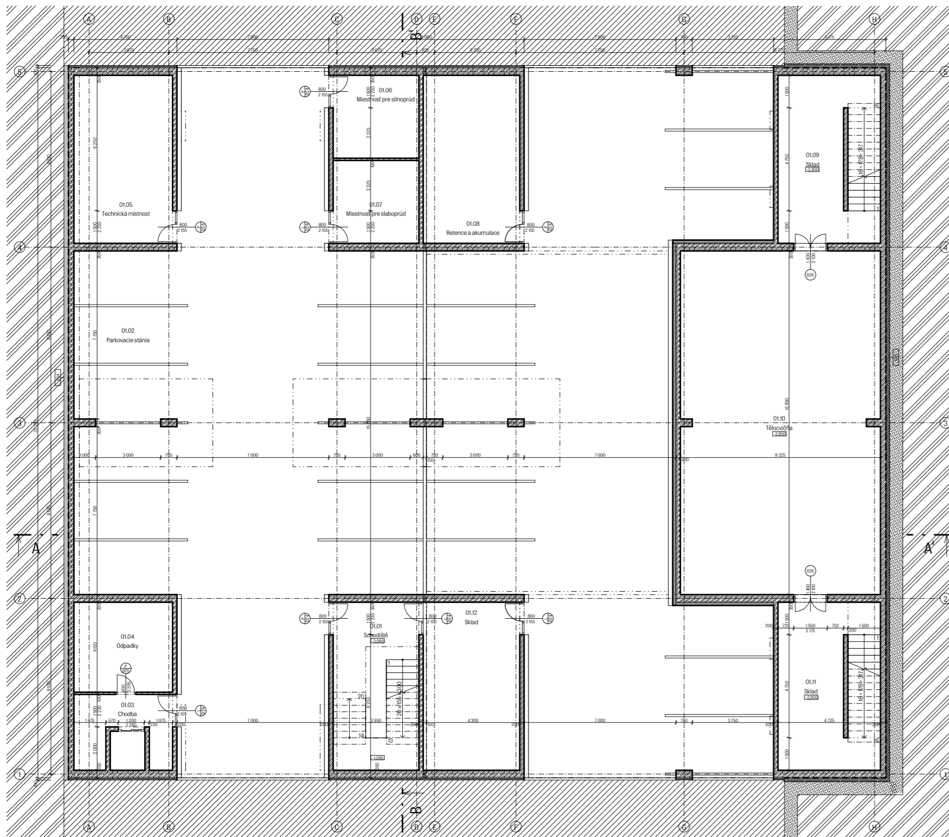
Legenda miestností a ploch 1.PP
