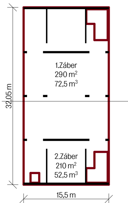
Zábery vodorovných konštrukcií M 1:400
