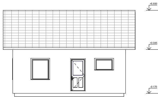
POHLED - VSTUP 1 : 50
