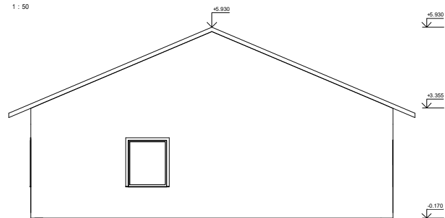
POHLED - BOČNÍ 1 : 50
