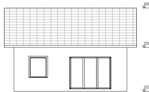
POHLED - ZAHRADA 1 : 50
