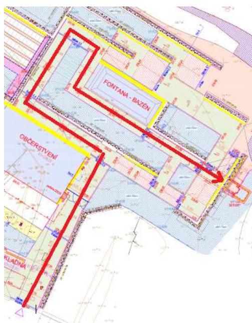
Obr. č. 2 - Nová trasa pro invalidy od parkovacího stání do výtahu-skleníku (Projektová dokumentace, 2013)
