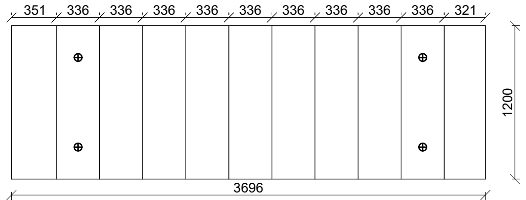
Pohľad spredu
