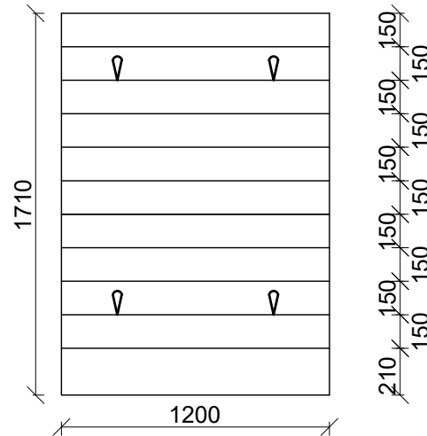
Pohľad spredu
