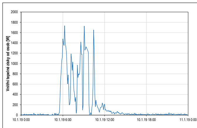
Obr. 10 Průměrné tepelné zisky od osob plynoucí z obsazenosti ve třídě Fig. 10 Average heat gains from people resulting from the class occupancy
