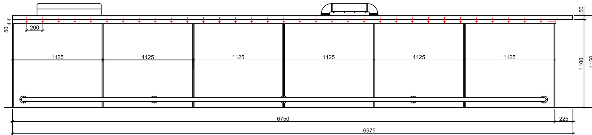
Východní pohled
