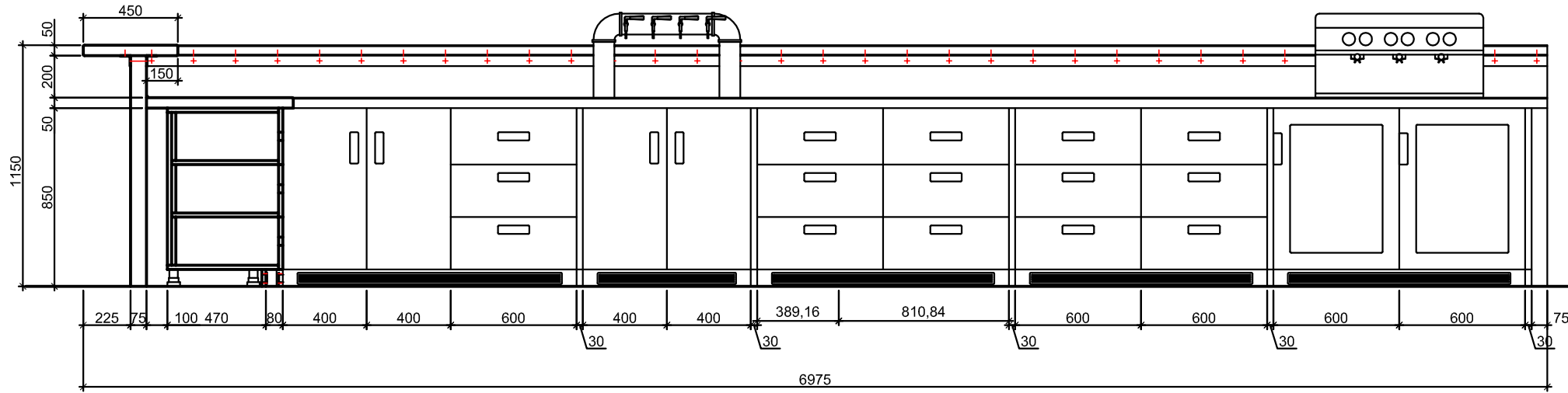
Západní řezopohled
