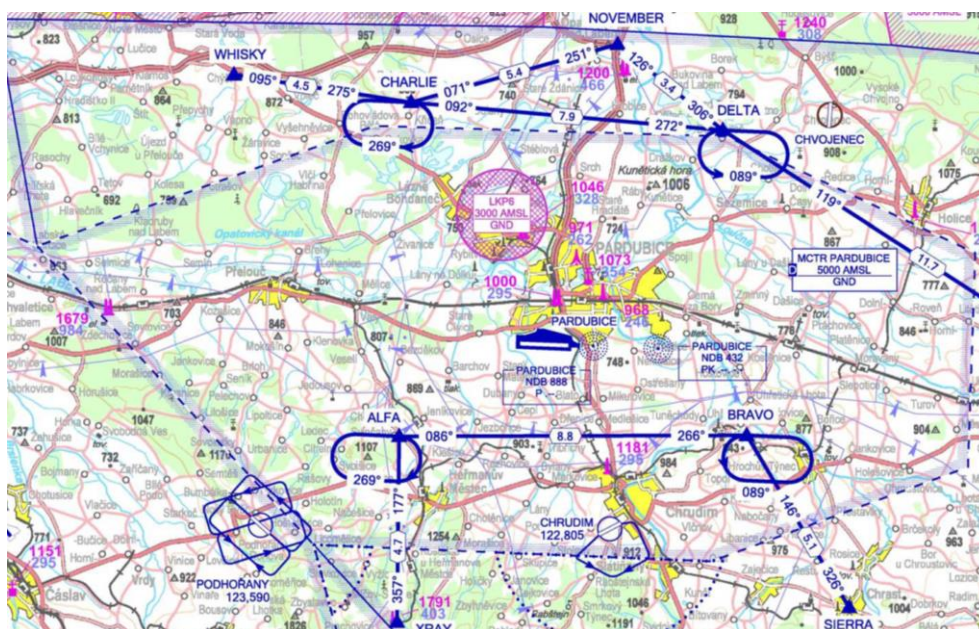
Obrázek 10. Poloha pardubického letiště vzhledem k městu (čárkovaně je vyznačena MCTR Pardubice) [28]
