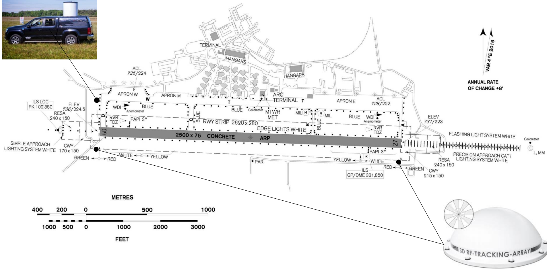
Obrázek 13. Rozmístění antén IsoLOG 3D DF-160 a mobilního systému ELVIRA na letišti Pardubice [28]
