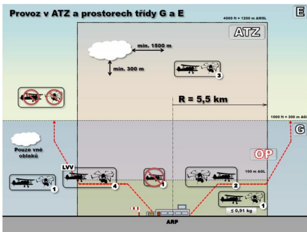
Obrázek 1. Provoz v ATZ a prostorech G a E [4]
