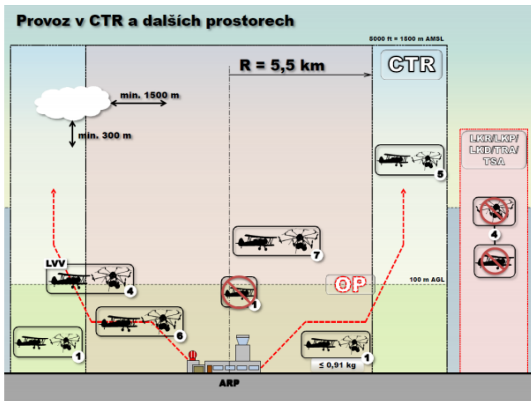
Obrázek 2. Provoz v CTR a dalších prostorech [4]
