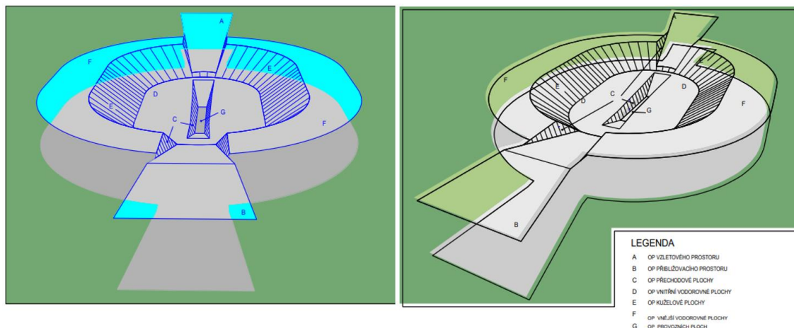
Obrázek 11. Ochranná pásma s výškovým omezením staveb pro přístrojovou ranvej [37]
