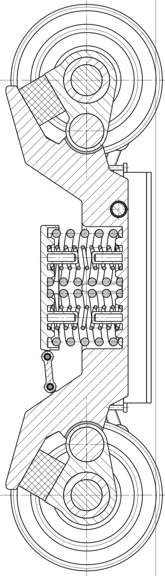
A-A (1:10)
