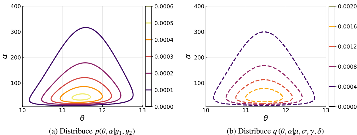
Obrázek 1.1: Contour plot distribuce p(\theta, \alpha | y_1, y_2) (vlevo plnou čarou) a q(\theta, \alpha | \mu, \sigma, \gamma, \delta) (vpravo čerchovaně), kde distribuce q je vyčíslena ve vypočtených odhadech \hat{\mu}, \hat{\sigma}, \hat{\gamma}, \hat{\delta} a distribuce p je vyčíslena v bodech y_1 = 11 a y_2 = 12 . Je patrné, že distribuce jsou téměř totožné.
