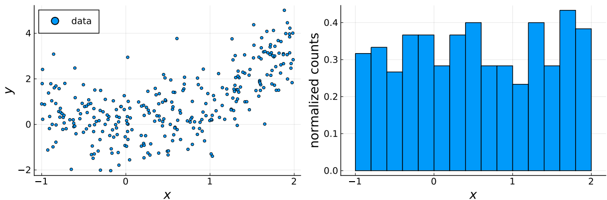
(a) Data, pro která hledáme distribuci p(x, y) .
