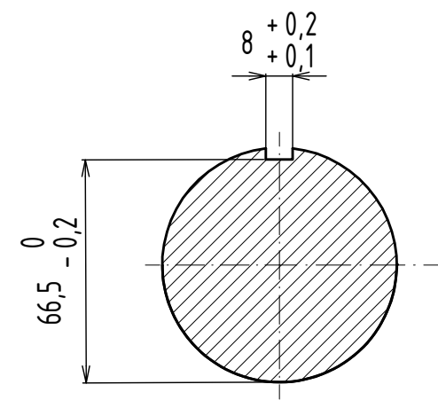
D-D (1:2)
