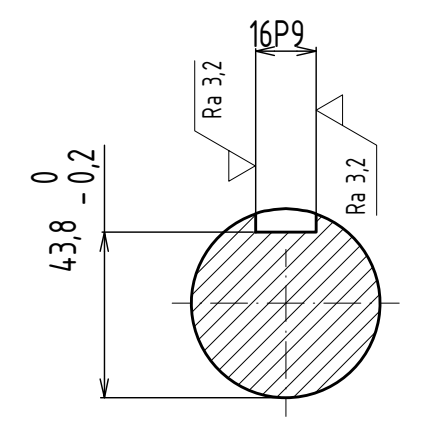
C-C (1:2)
