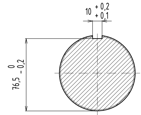
B-B (1:2)
