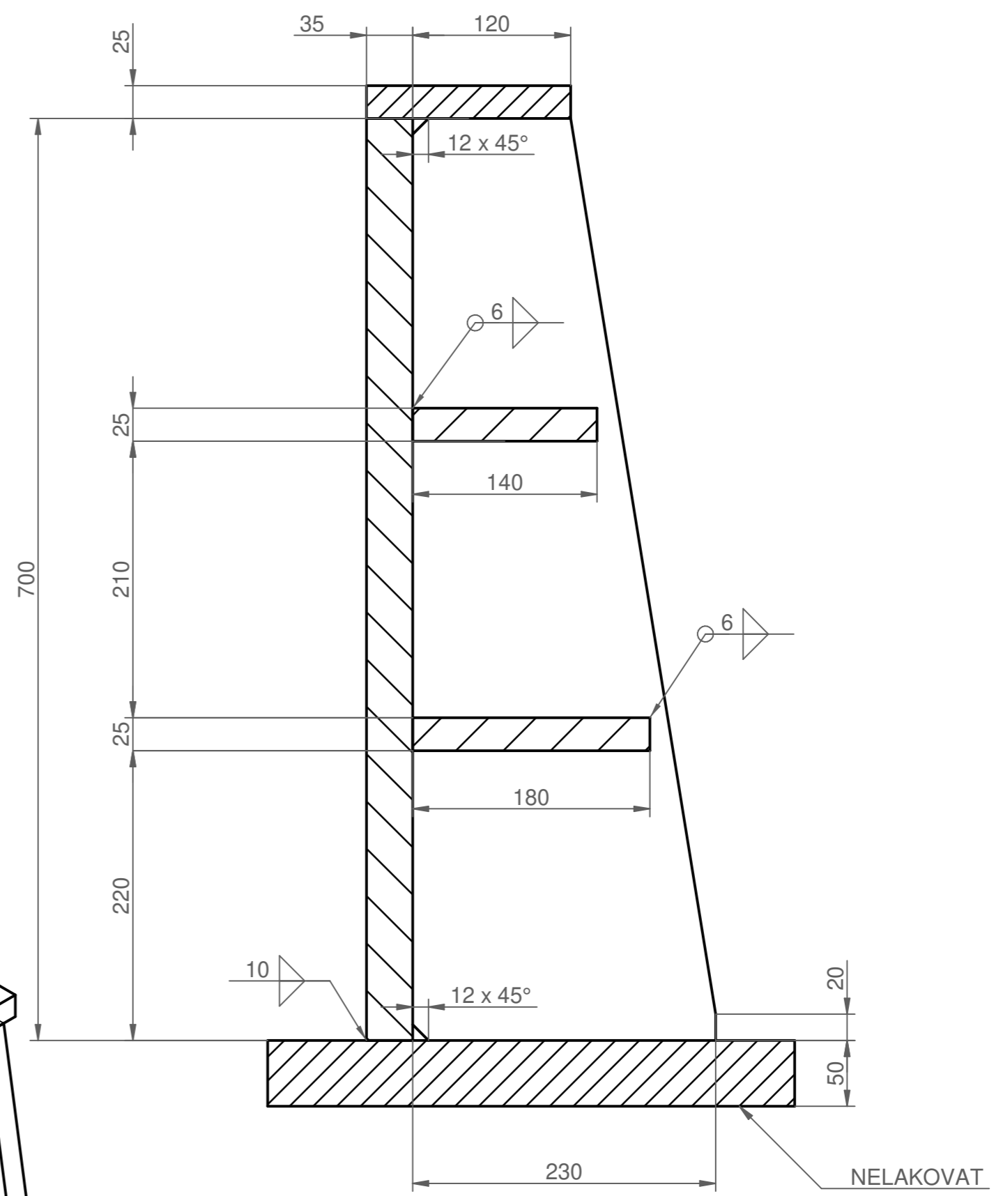
Řez A-A
