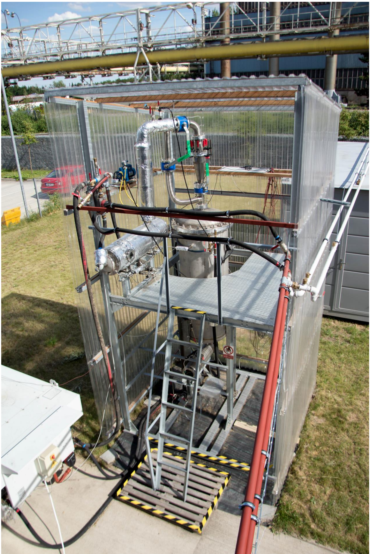
Pilotní jednotka s absorpčním oběhem pro produkci práce
