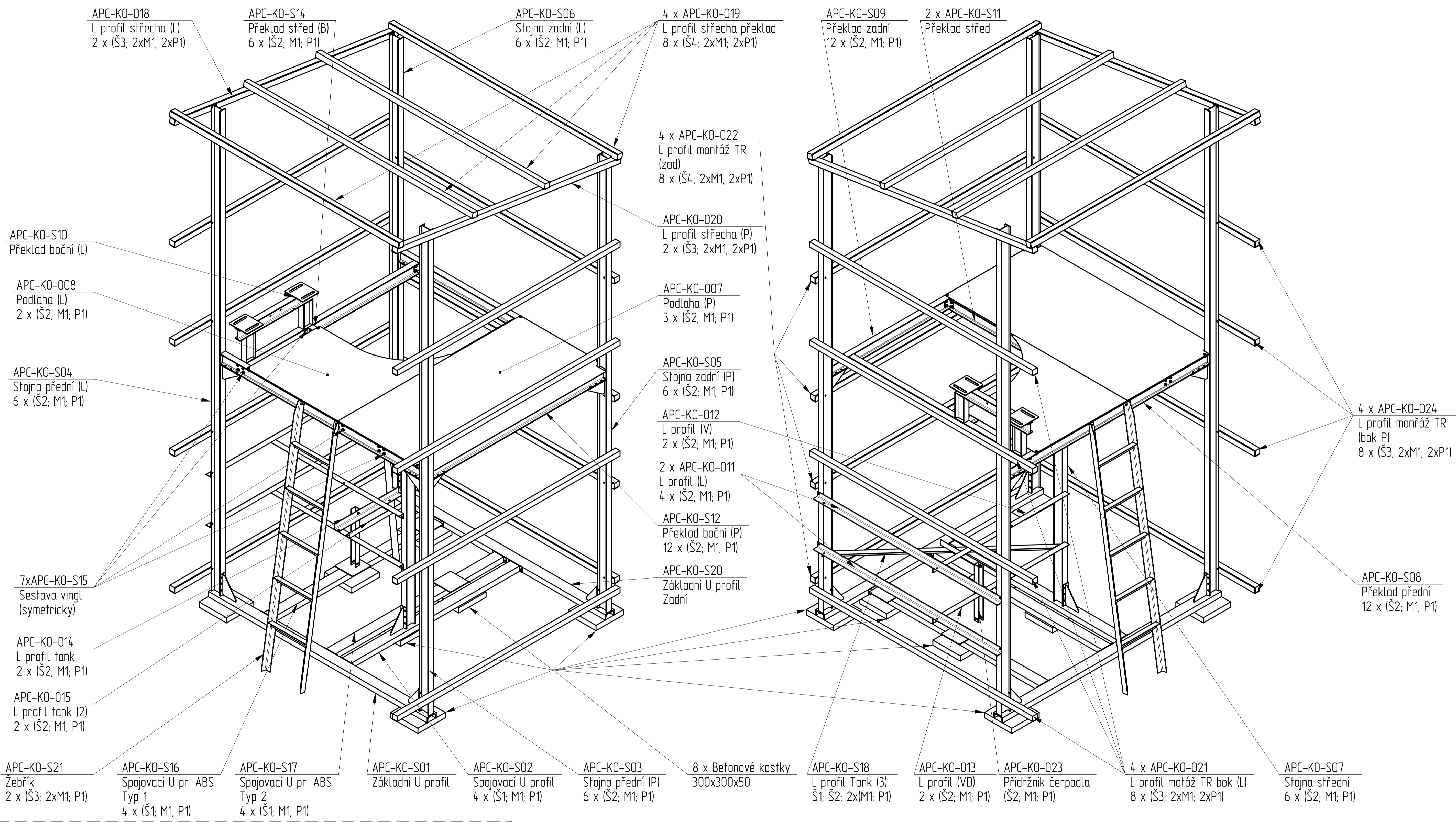
DETAIL střecha bok
