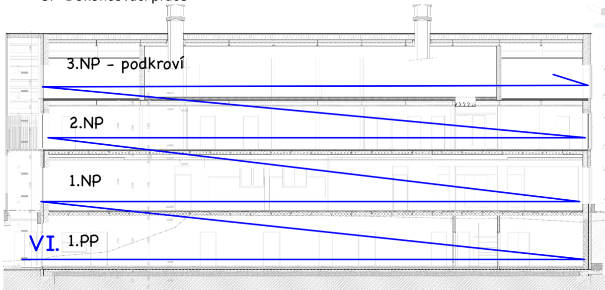
Obr. 12 - Směr postupu výstavby pro etapu VI. [vlastní tvorba]
