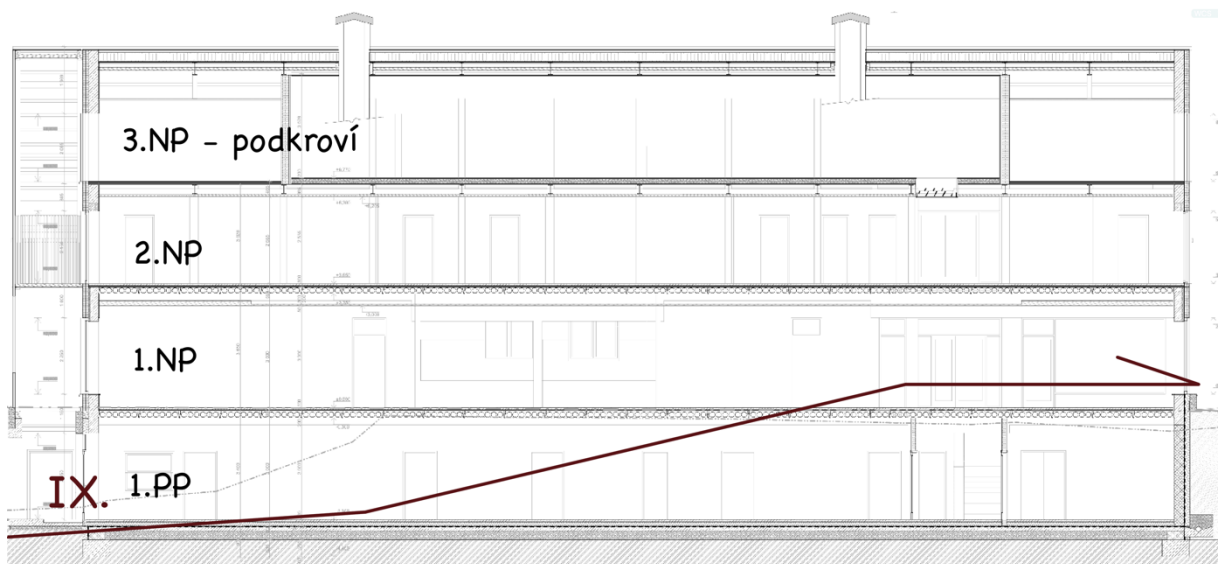
Obr. 15 - Směr postupu výstavby pro etapu IX. [vlastní tvorba]
