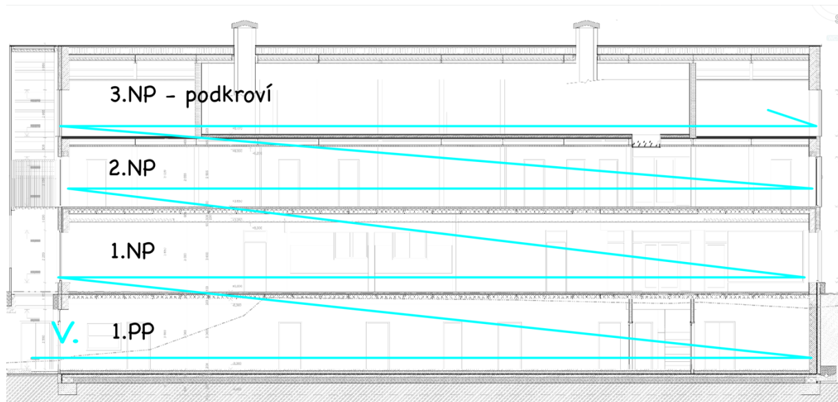
Obr. 11 - Směr postupu výstavby pro etapu V. [vlastní tvorba]
