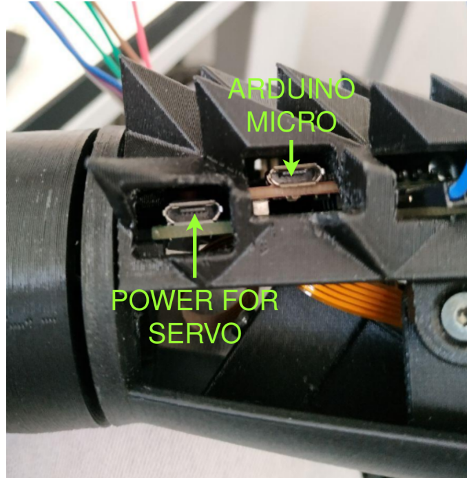
Obrázek A.3: Připojení robotické ruky
