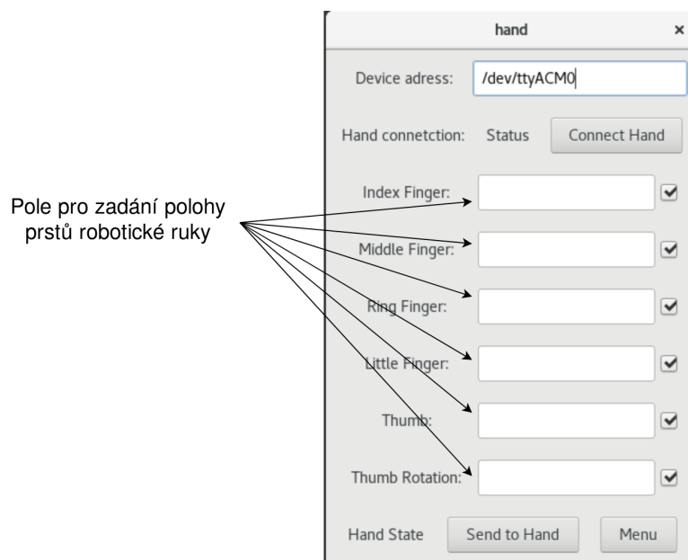
Obrázek 5.12: Obrazovka manuálního ovládání
