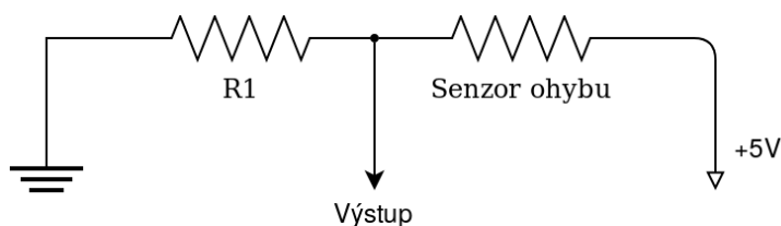
Obrázek 5.6: Připojení senzoru ohybu
