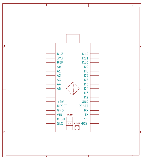
Obrázek 2.4: Arduino Micro
