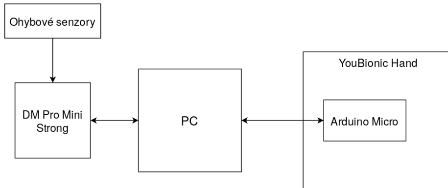
Obrázek 4.6: Navrhované schéma modelu
