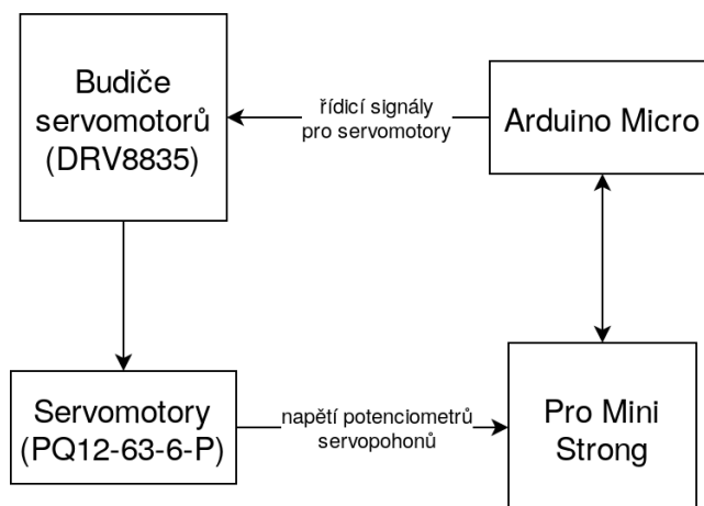
Obrázek 4.1: Komunikace komponent robotické ruky
