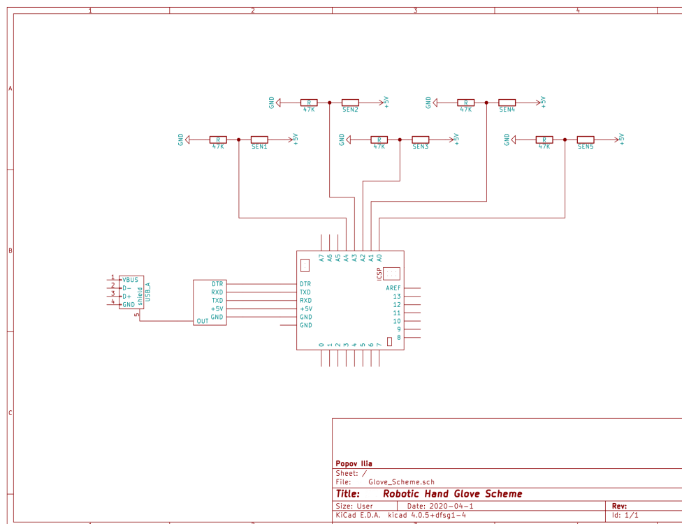
Obrázek 5.7: Schéma zapojení rukavice
