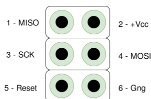
Obrázek 4.3: ICSP
