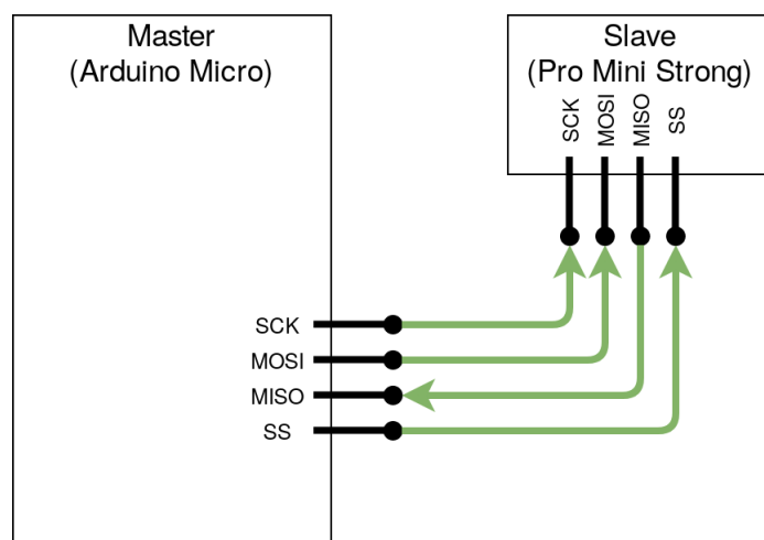
Obrázek 4.2: SPI komunikace
