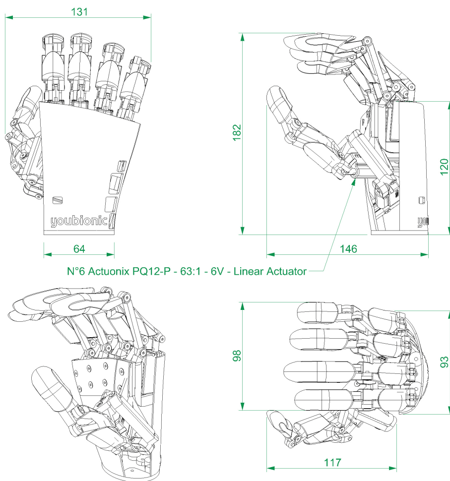
Obrázek 2.1: Youbionic Hand. Převzato z [1].
