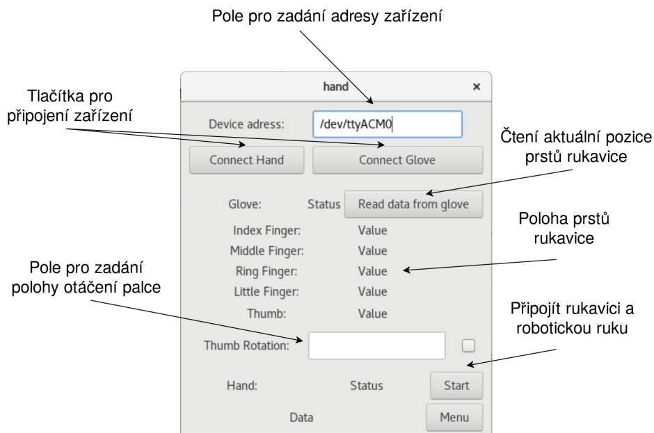
Obrázek 5.11: Obrazovka ovládání přes rukavice
