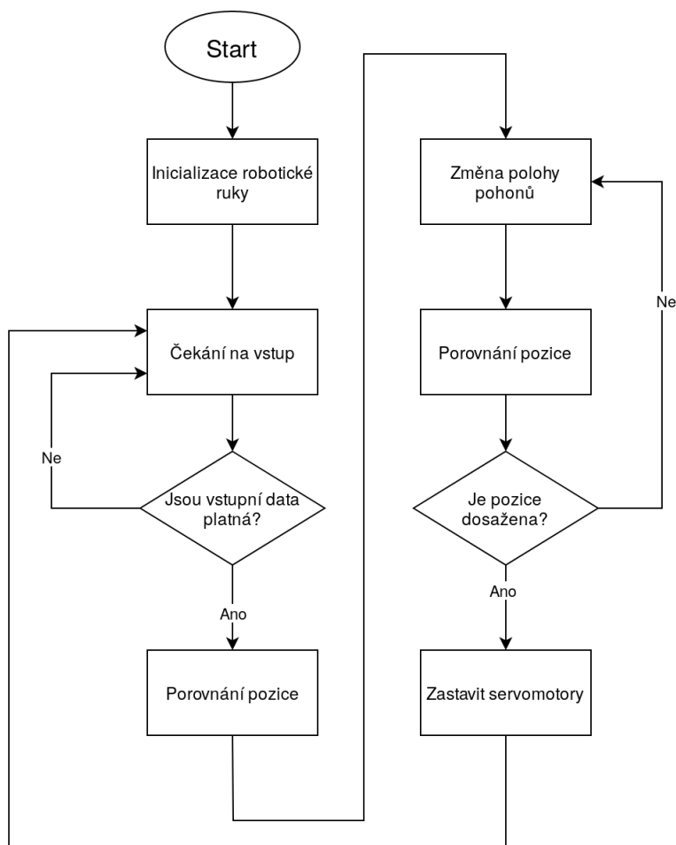
Obrázek 5.8: Program pro hlavní řídicí jednotku robotické ruky
