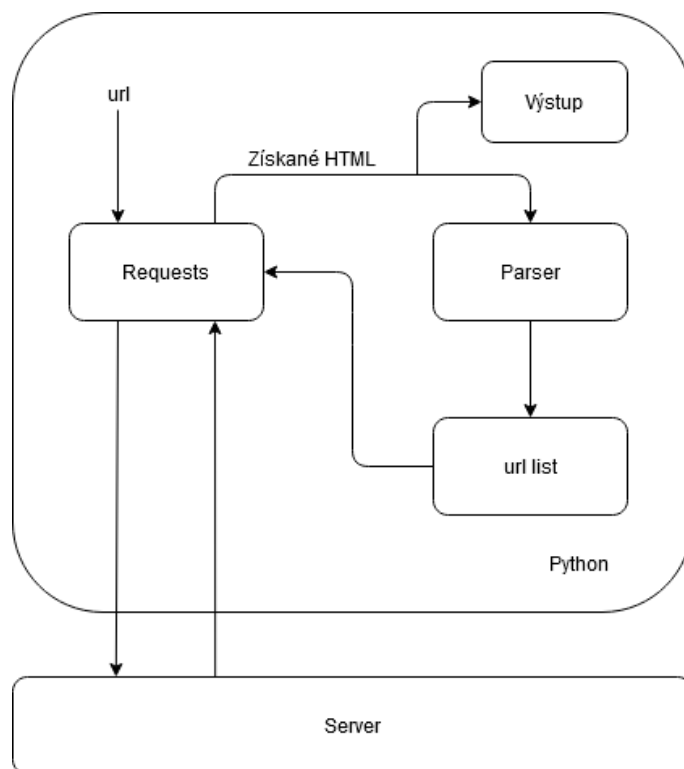
Obrázek 2.1: Diagram zachytávání komunikace pomocí web scrapperu
