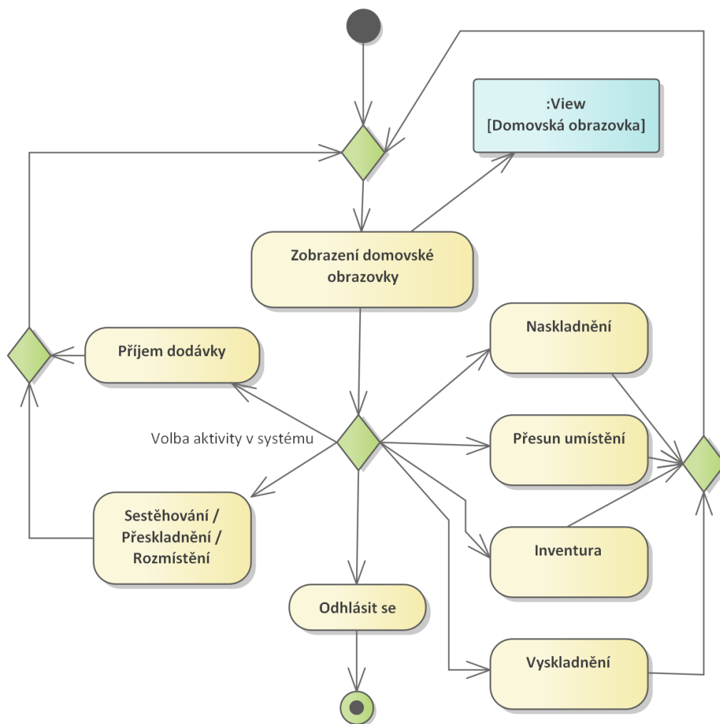
Obrázek C.1: Activity diagram průchodu systémem skladníkem: první část
