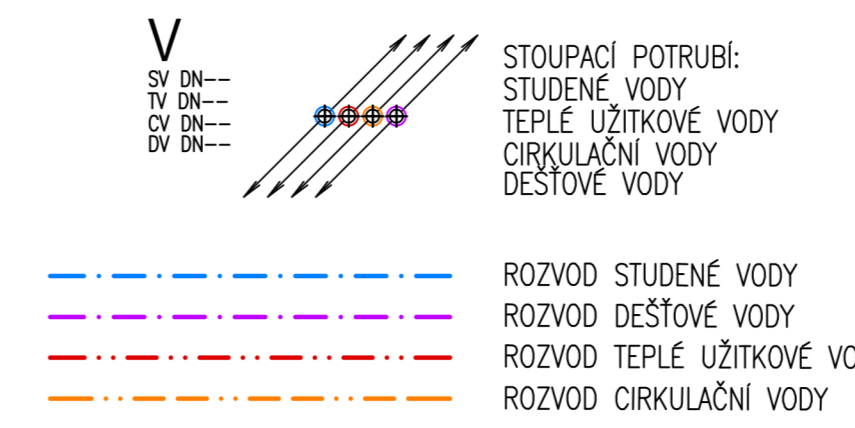
LEGENDA VODOVODU:
