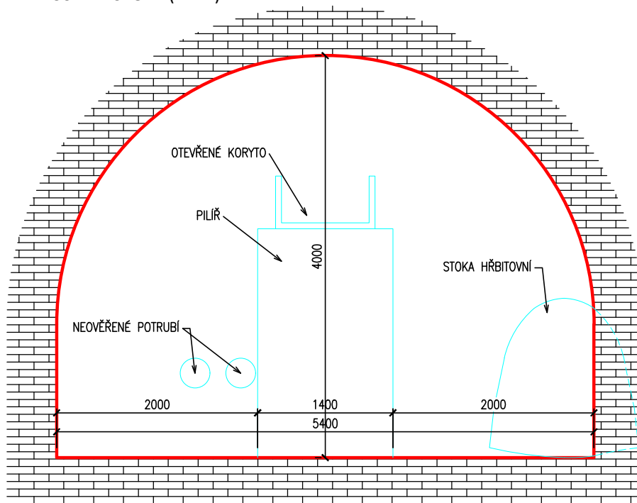
PORTÁL VYÚSTĚNÍ STOKY (HB-V)
