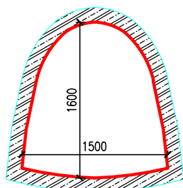
TYP PROFILU - P1
