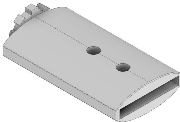
Obr. 4 Pouzdro listu rotoru
