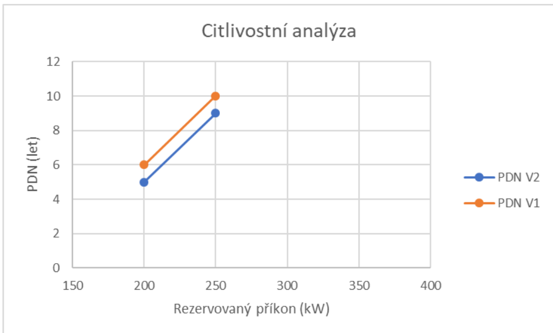
Graf 9 Citlivostní analýza – Prostá doba návratnosti
