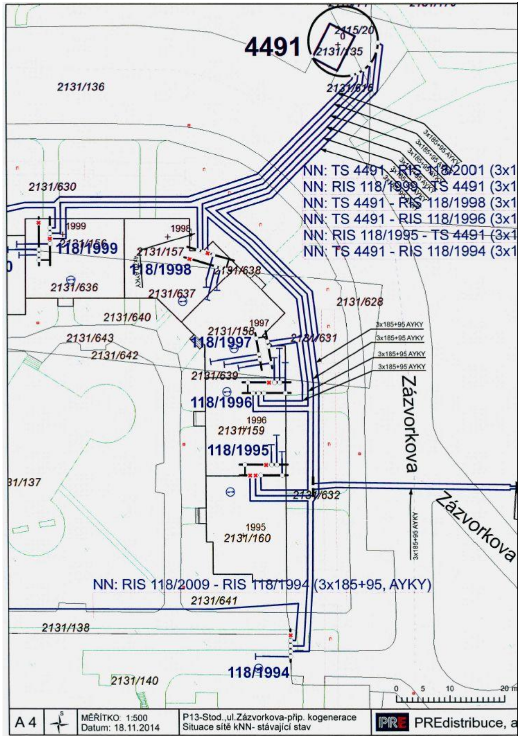
Obr. 3 Připojení objektu
