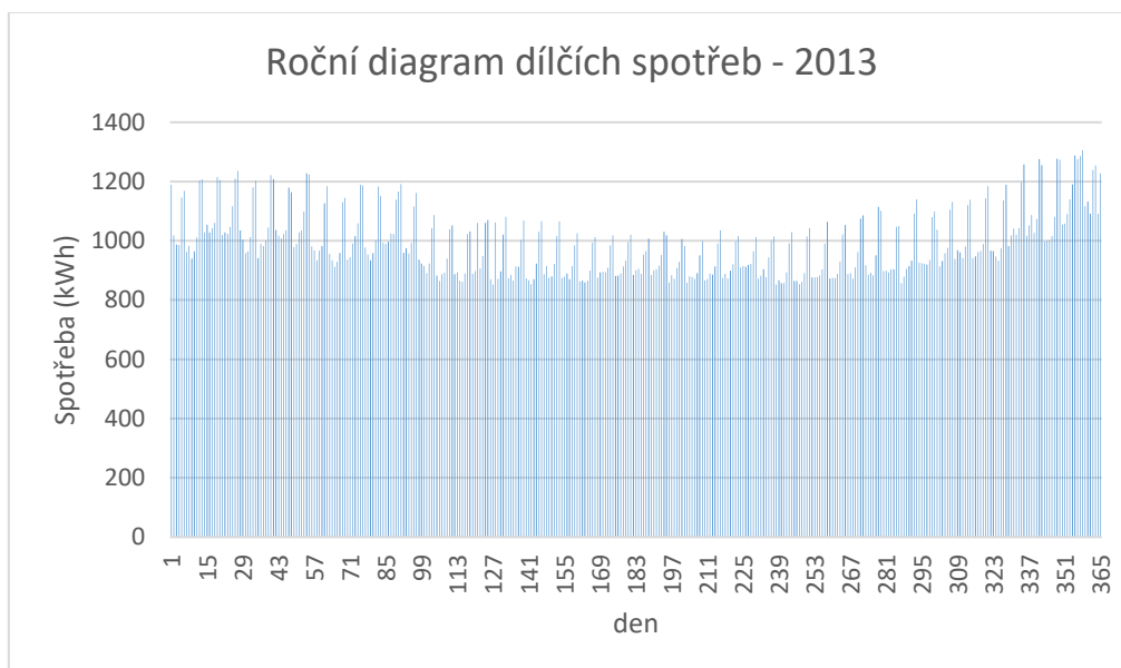
Graf 5 Roční diagram dílčích spotřeb – 2013
