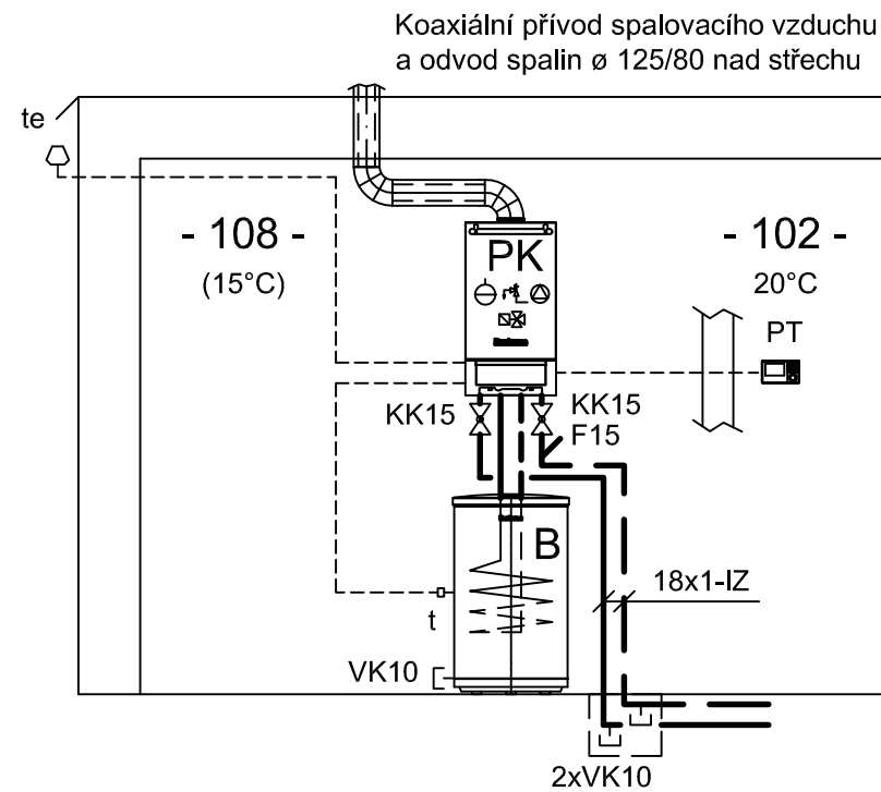
Půdorys 1. NP
