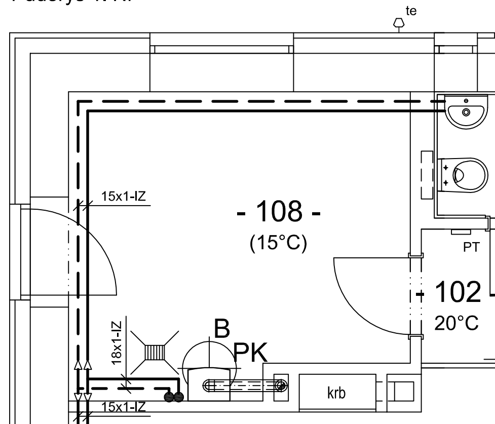
Půdorys 1. NP
