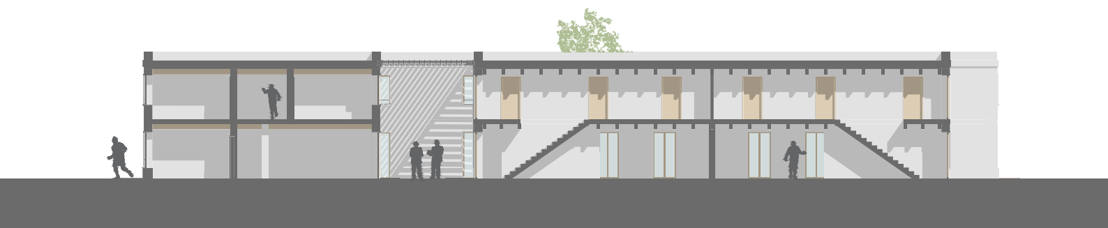
řez D-D'
