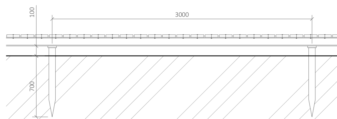
2 POCHOZÍ LÁVKA POHLED M 1:25
