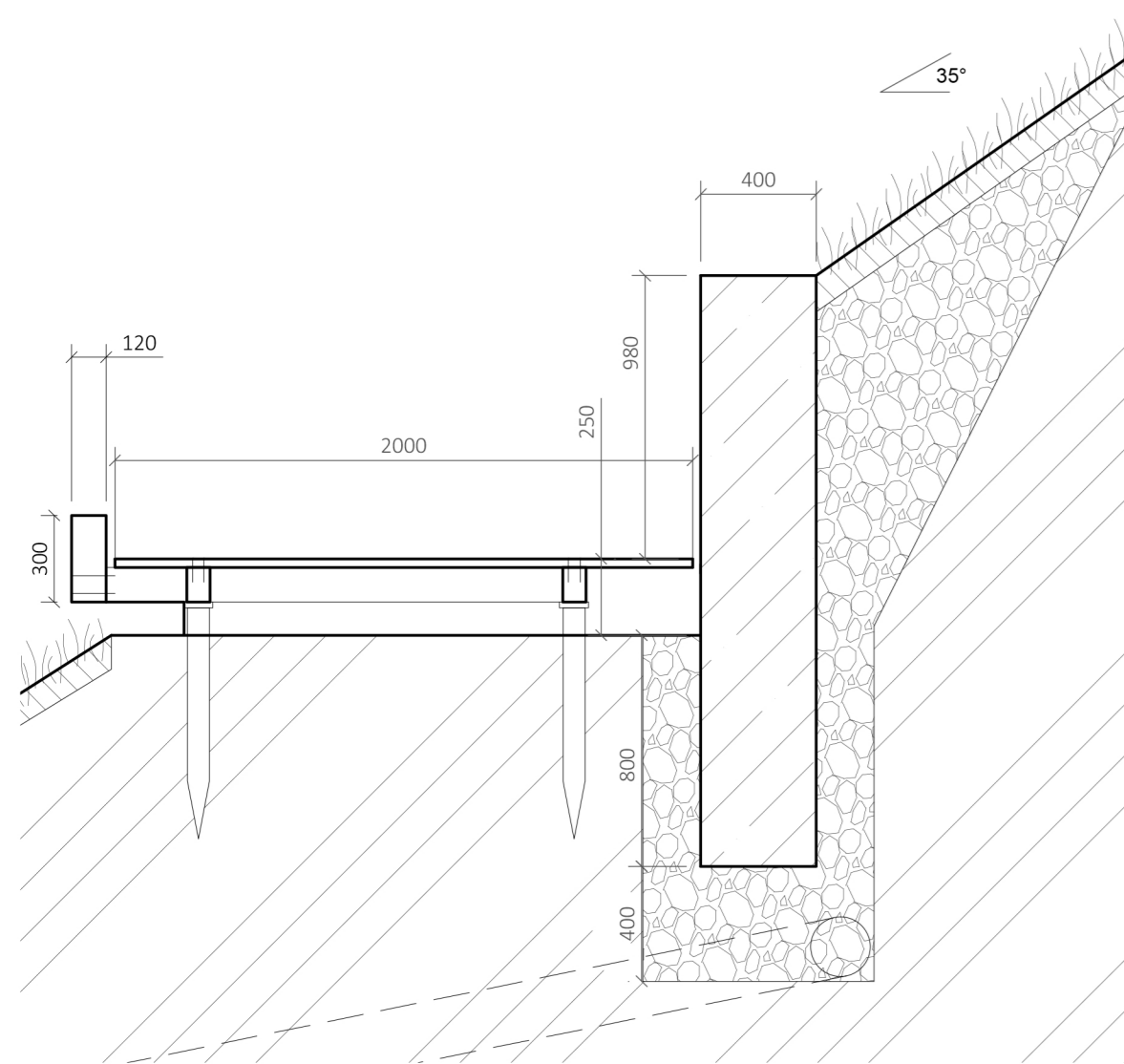
2 POCHOZÍ LÁVKA POHLED M 1:25
