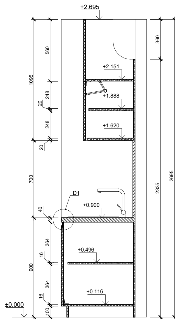
ŘEZ B-B'
