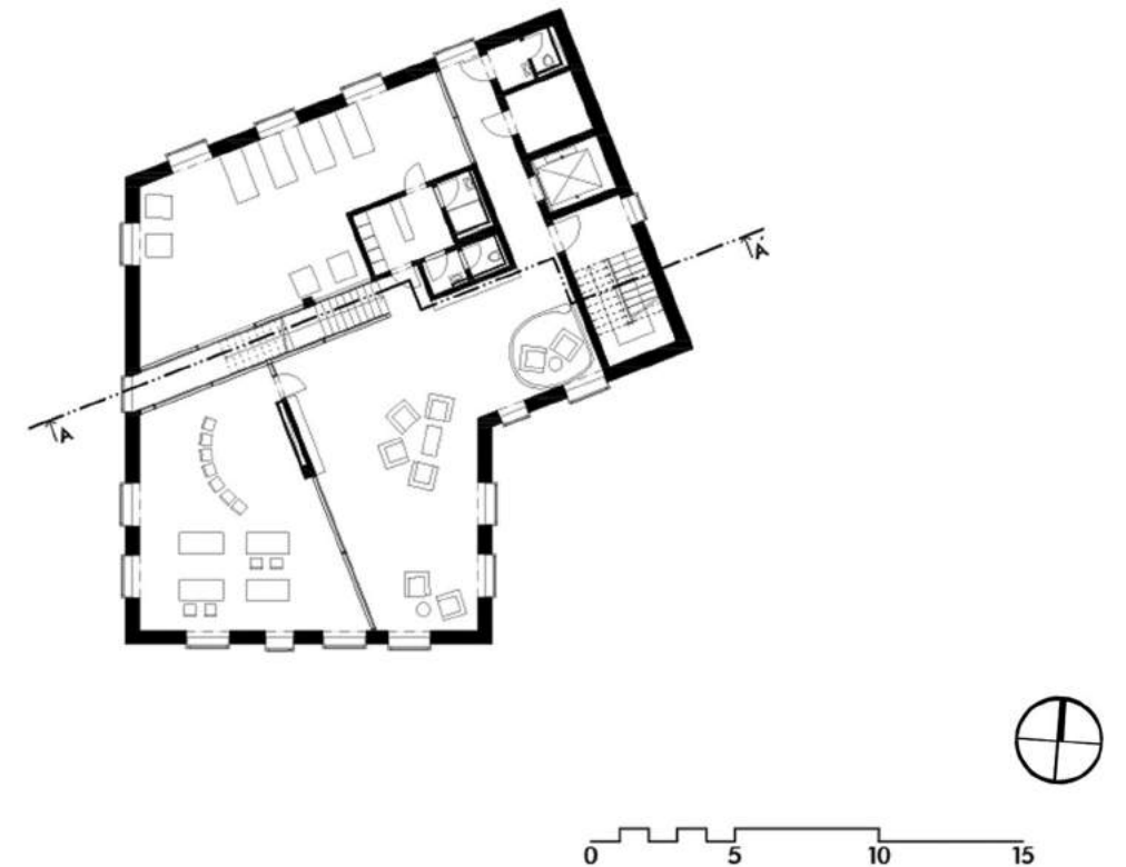
PŪDORYS 3.NP
