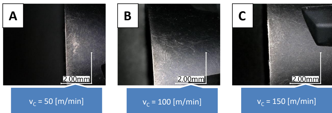
Obr. 56 Opatření hřbetu nástroje – RPHX 1204M4EN-M32
