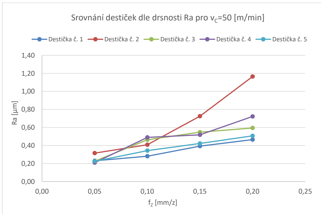
Obr. 70 Srovnání destiček dle drsnosti obrobene plochy
