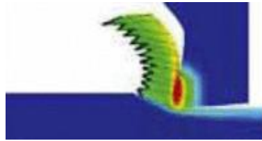
Obr. 12 Vznik smykových pásem u obrábění titanu [12]
