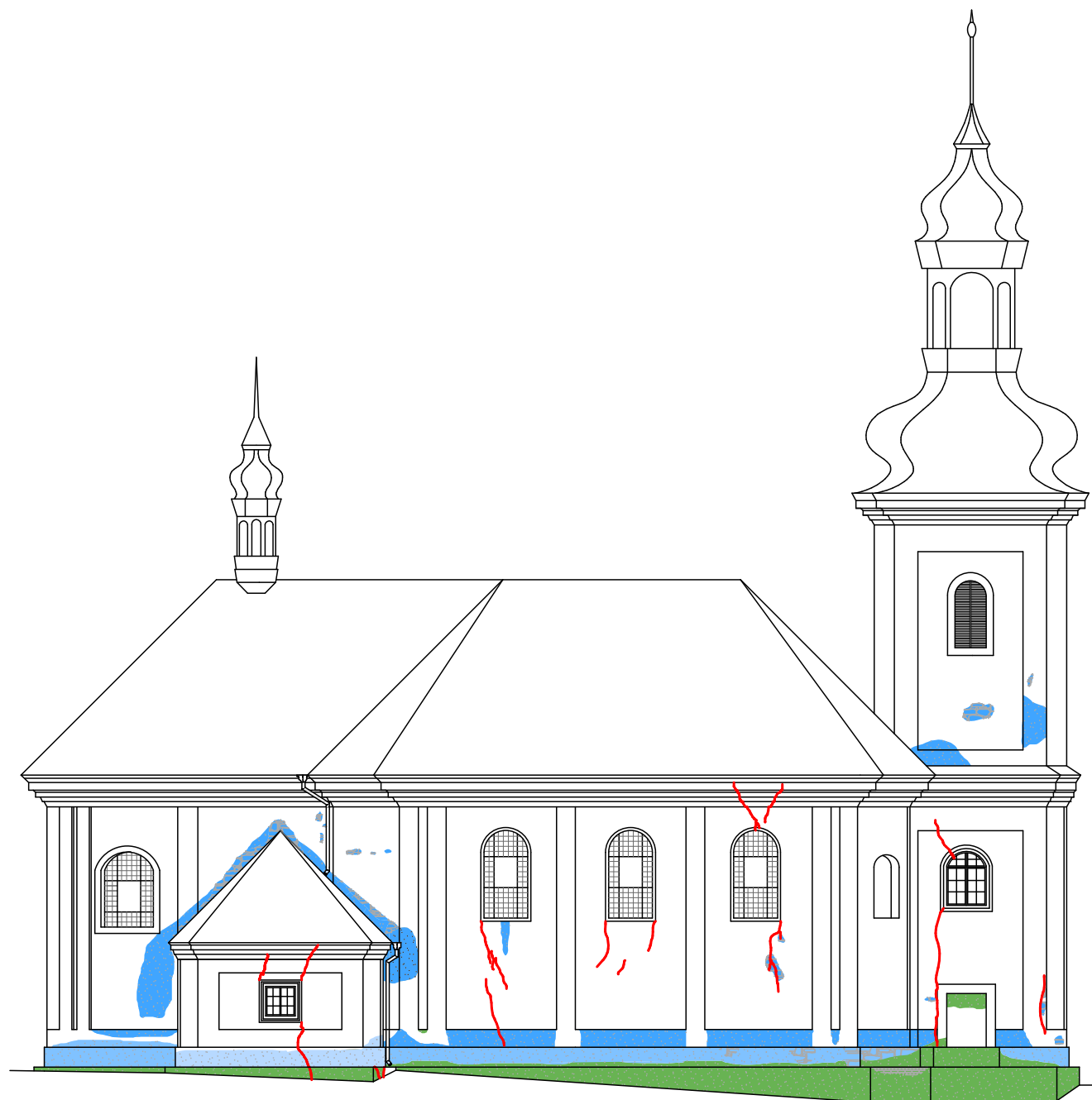
POHLED SEVERNÍ
