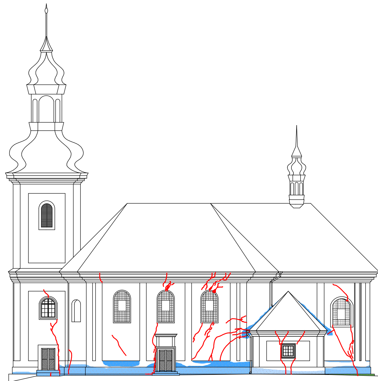
POHLED JIŽNÍ
