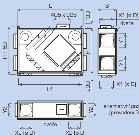
PODSTROPNÍ (pohled shora) Basic 1 400 až 8 100
