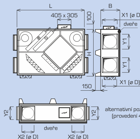
PODLAHOVÁ (pohled shora) Basic 1 400 až 8 100
