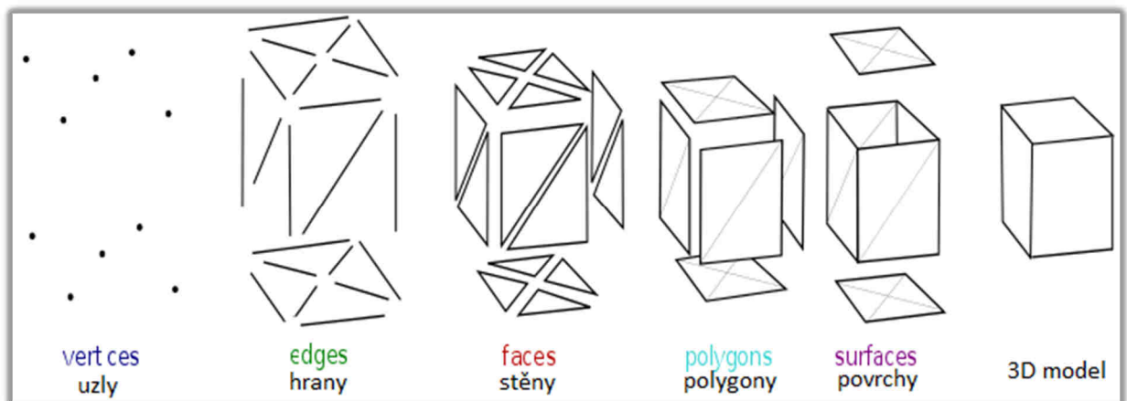
Obrázek 28 - Proces tvorby 3D modelu [wikipedia.org]
