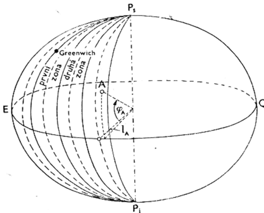
Obrázek 14 - Gauss-Krügerovo zobrazení [ http://old.gis.zcu.cz/ ] 18
