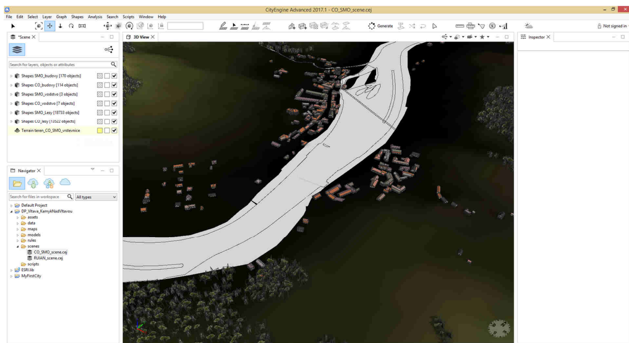
Obrázek 6 - CityEngine
