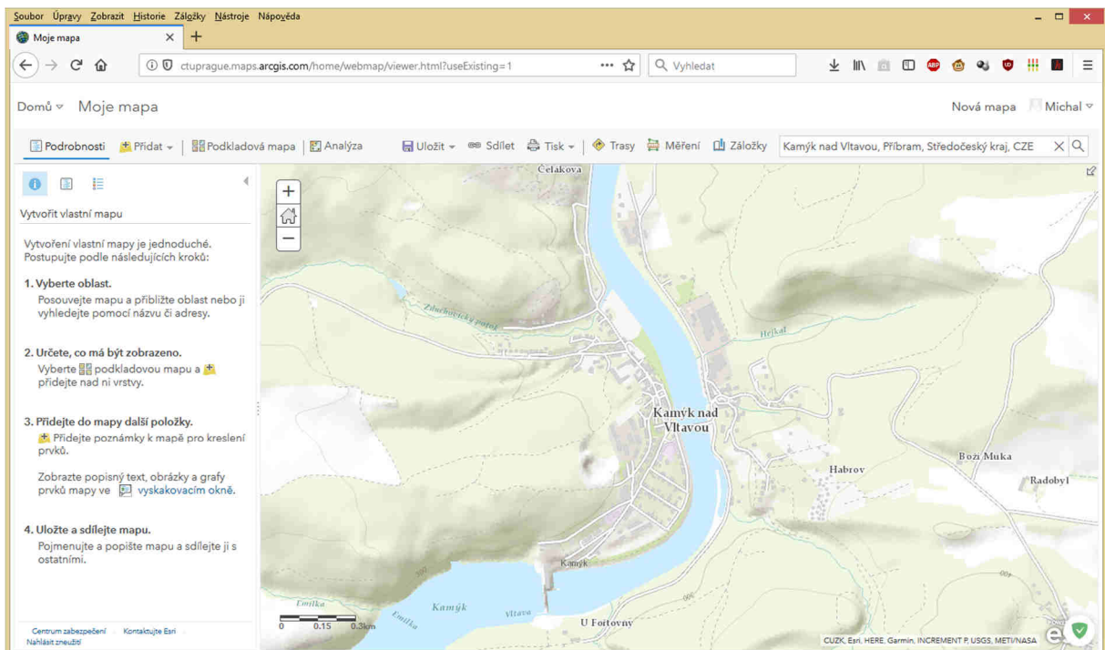
Obrázek 5 - ArcGIS Online
