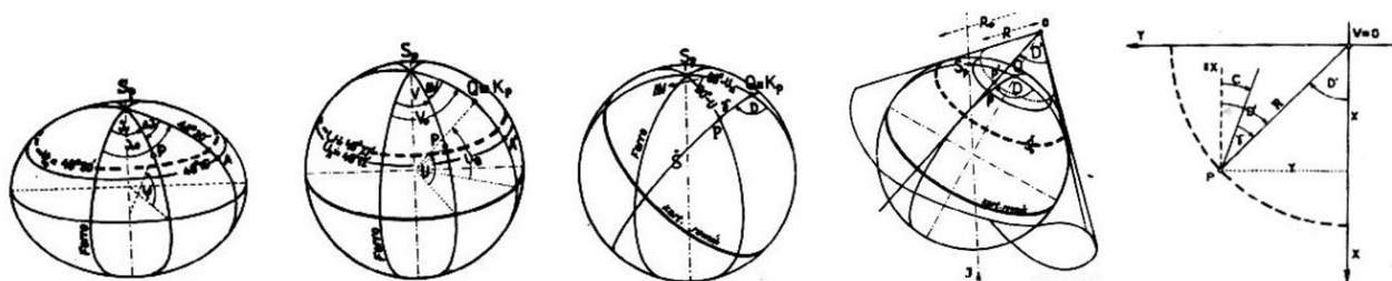
Obrázek 11 - Transformace v krocích - elipsoidické, sférické, kartografické, polární a rovinné souřadnice
