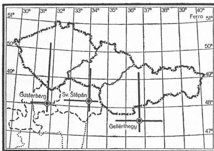
Obrázek 9 – Souřadné systémy stabilního katastru [Opálková, T.] 13
