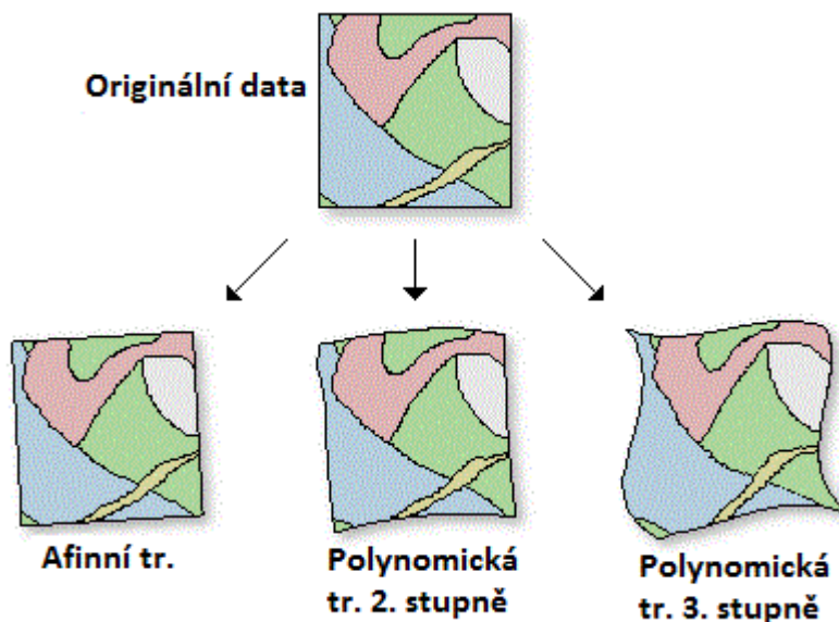
Obrázek 20 - Zobrazení rozdílů polynomických transformací [upraveno podle https://pro.ArcGIS.com/ ] 25
