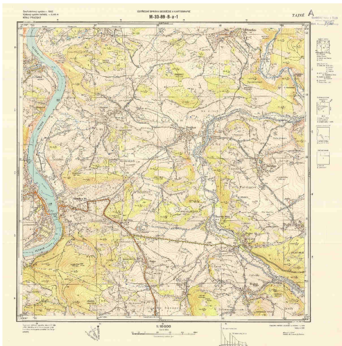
Obrázek 13 - Topo mapa v systému S-1952, 1 : 10 000, M-33-89-B-a-1
