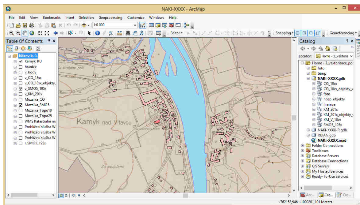
Obrázek 4 - ArcMap
