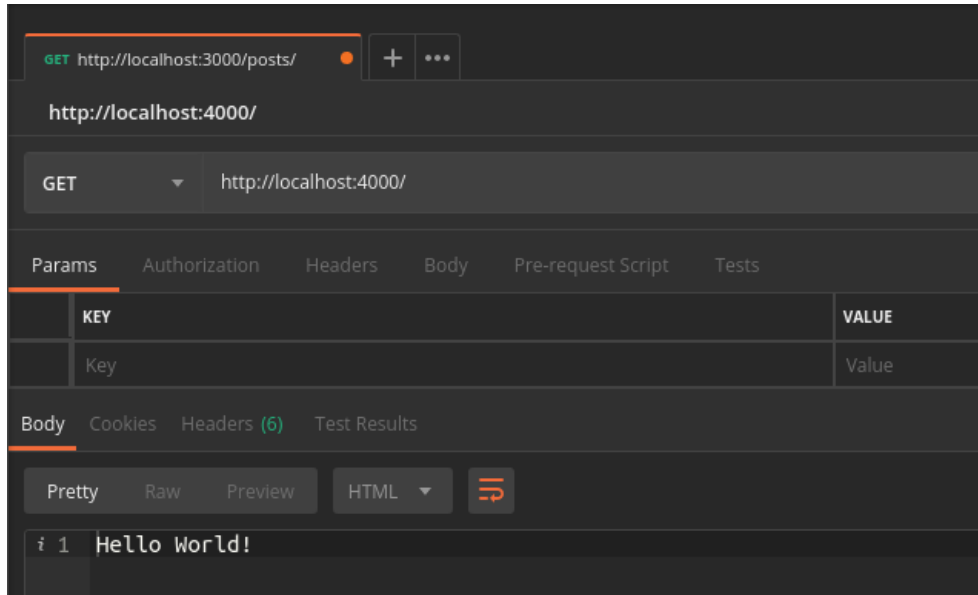
Obrázek 4.1: Postman
