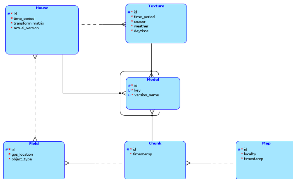
Obrázek 3.2: Současná databáze
