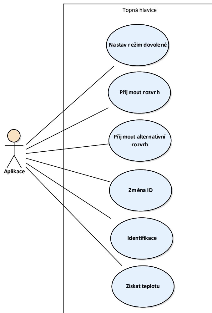
Obrázek 4.4: Diagram užití – Komunikace aplikace s hlavicí
