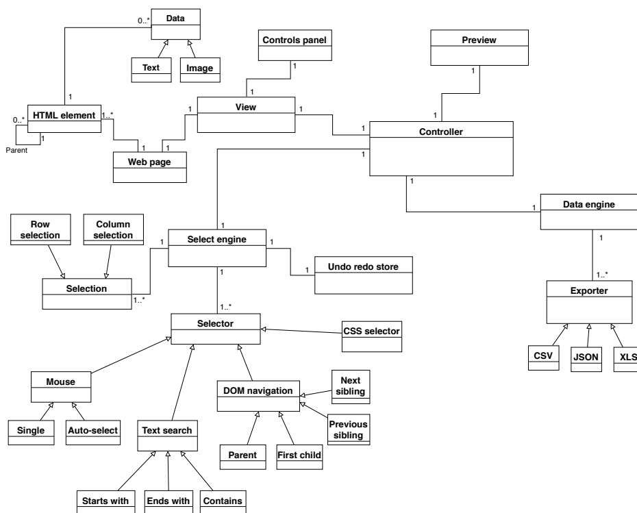
Obrázek 2.1: Diagram představující analytický doménový model
