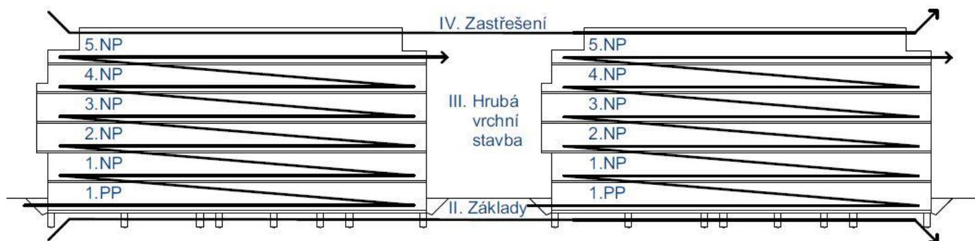
Obr. č. 15 – Směr postupu výstavby pro etapy II, III a IV
