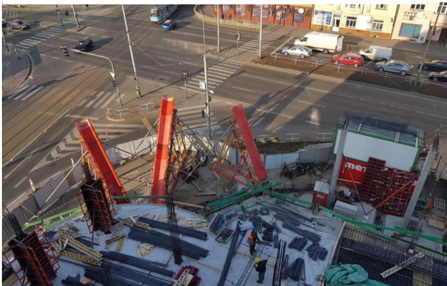
Obr. 2: Posun oplocení kvůli betonáži šikmých sloupů (vlastní zdroj)
