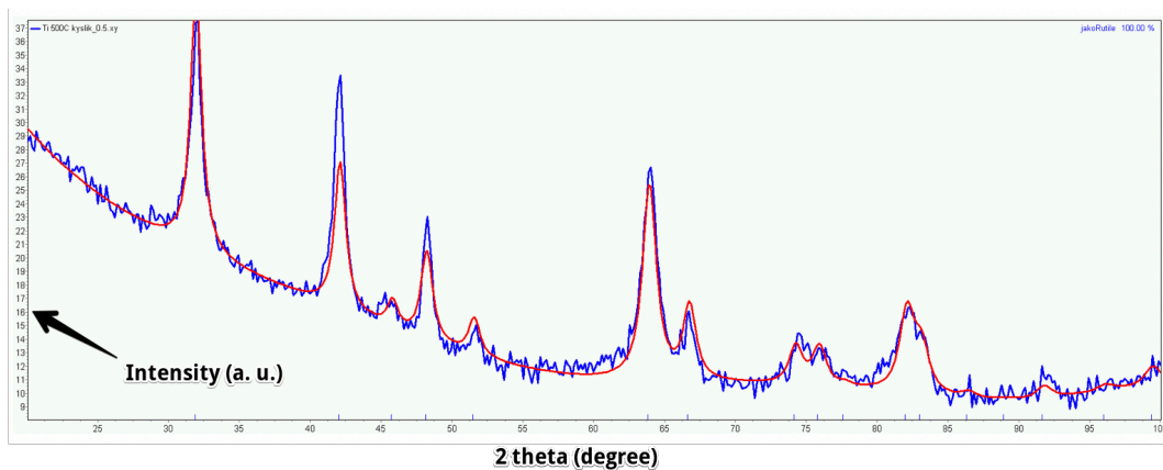
Obr. 34: Analýza XRD vzorku 500
