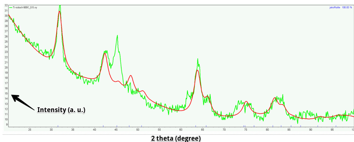
Obr.35: Analýza XRD vzorek 600
