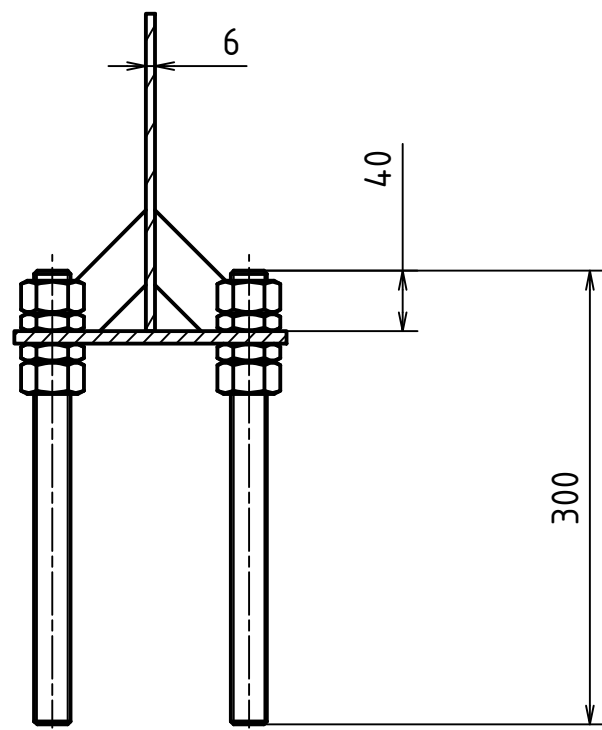
A-A (1:5)
