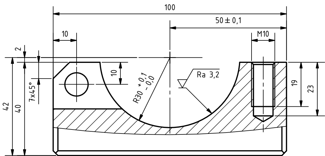
ŘEZ A-A
