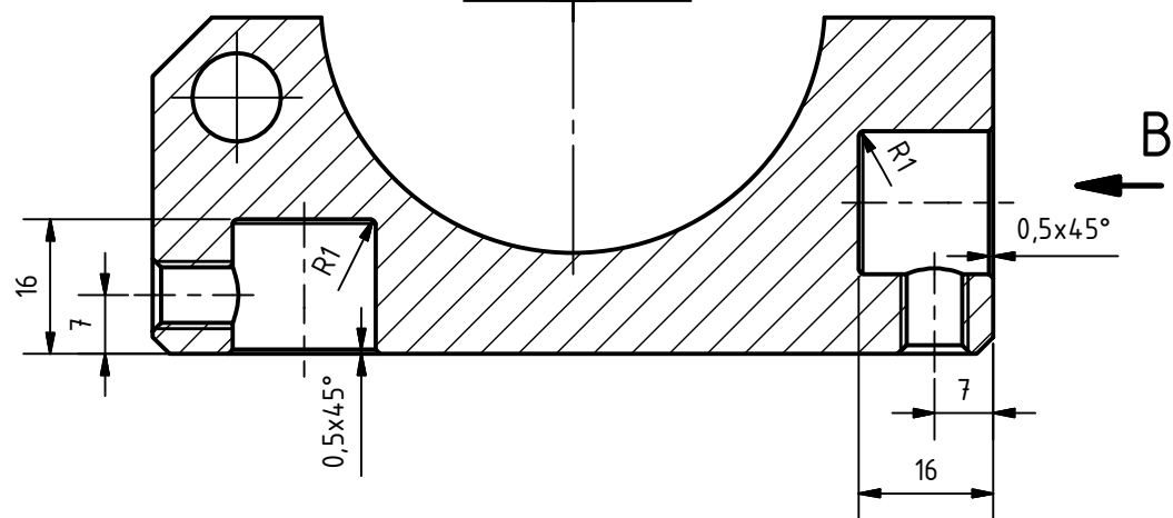
ŘEZ A-A
