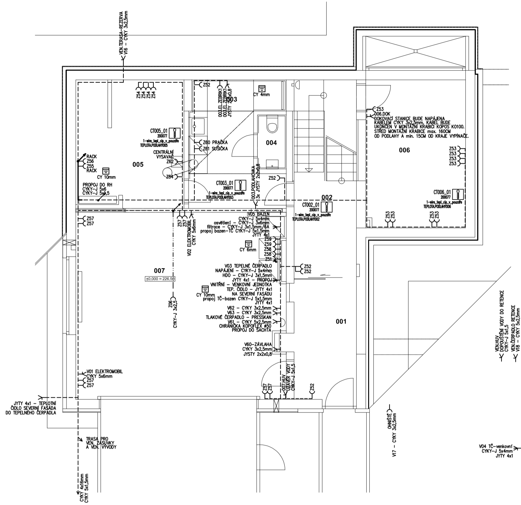
PŮDORYS 1. PP - ŘEZ ÚROVNÍ -1,000
