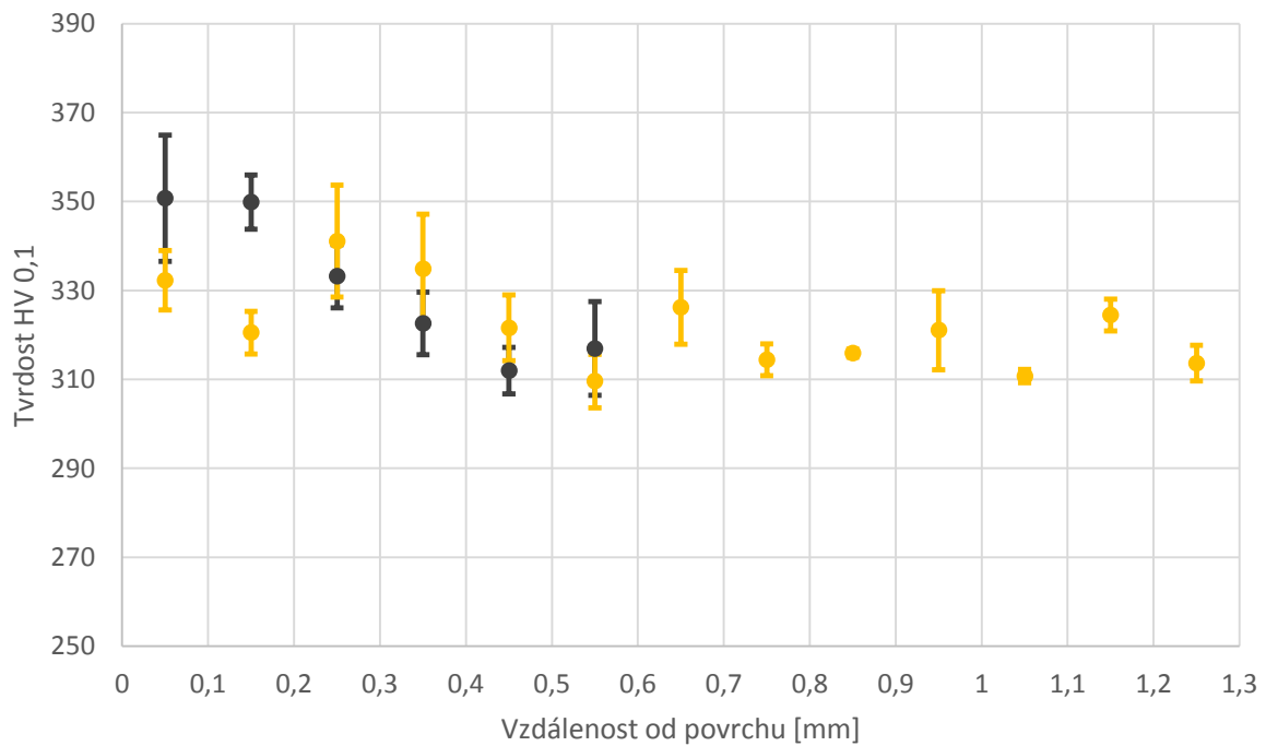
Tvrdość HV 0,1 při 2500 pulzech /cm 2
