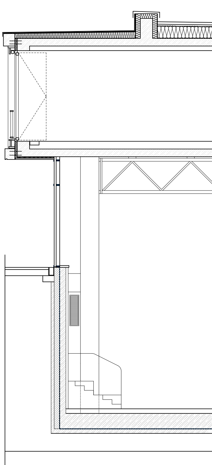
Řez fasádou M 1:75
