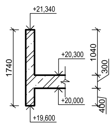
ŘEZ 5-5'
