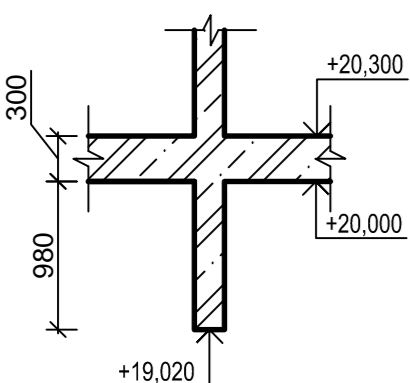
ŘEZ 10-10'
