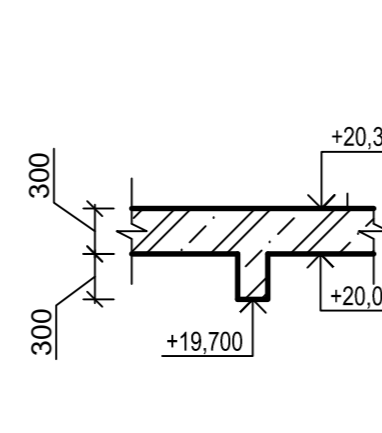
ŘEZ 3-3'
