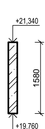
ŘEZ 2-2'
