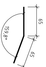
délka 2645 pohledová strana roh 1ks
