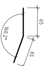
délka 2645 pohledová strana roh 1ks
