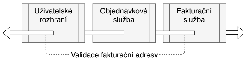
Obrázek 2.3: Příklad funkcionality zasahující do více služeb
