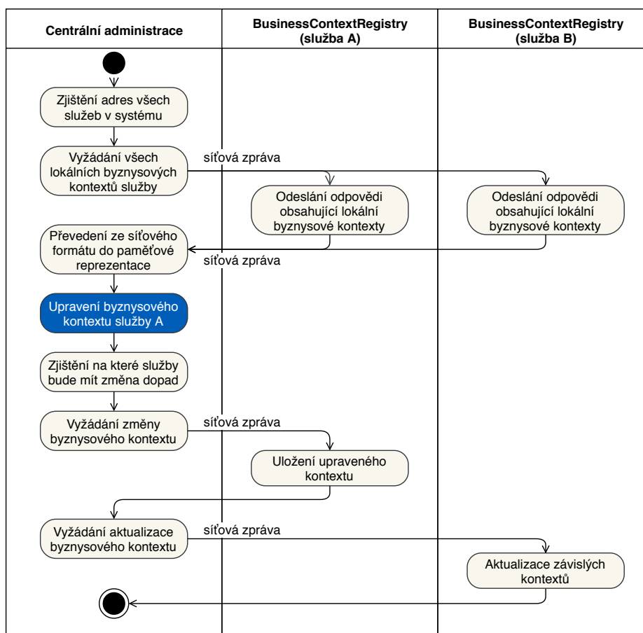
Obrázek 4.7: Proces centrální správy byznysových kontextů
