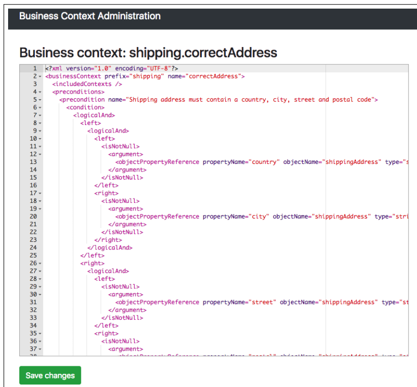
Obrázek B.2: Formulář pro vytvoření nebo úpravu byznysového kontextu v centrální administraci
