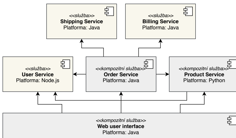
Obrázek 6.2: Komponenty ukázkového e-commerce systému
