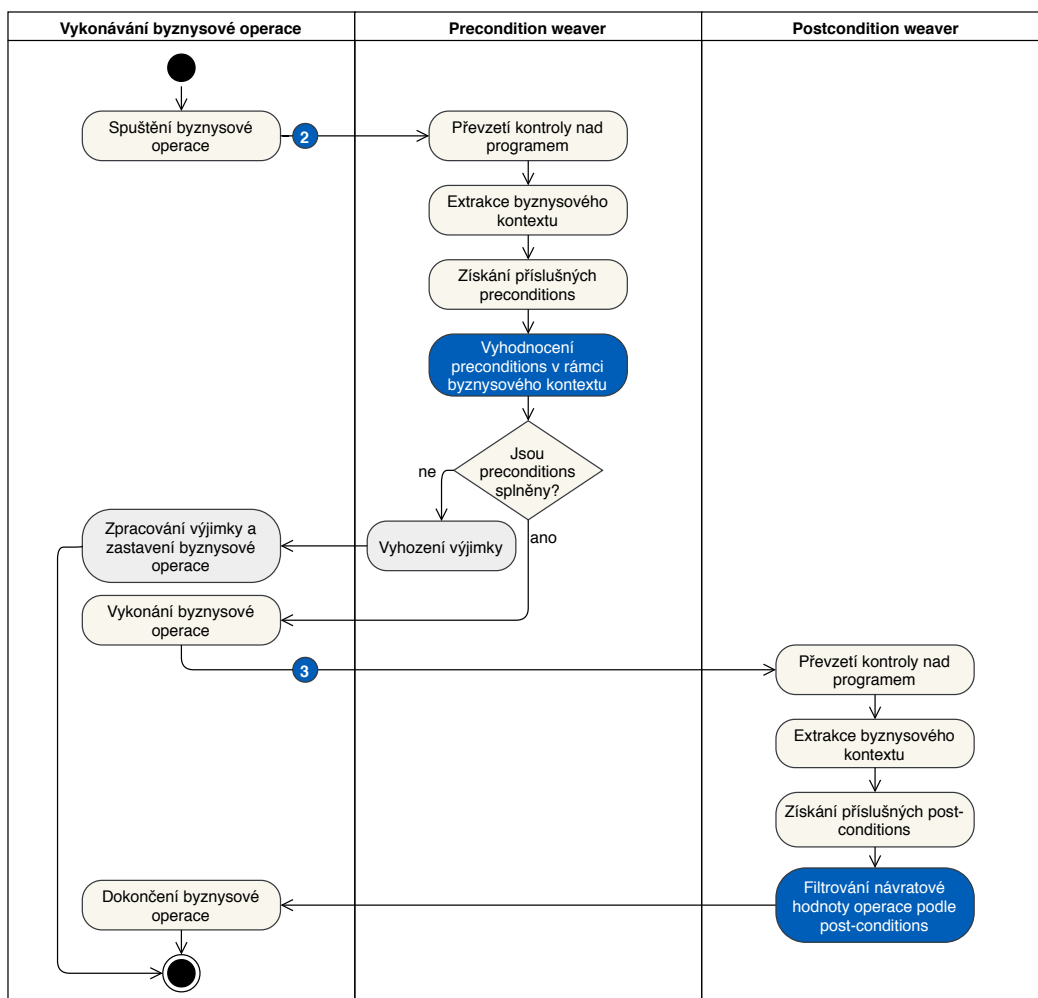
Obrázek 4.2: Proces weavingu byznysových pravidel
