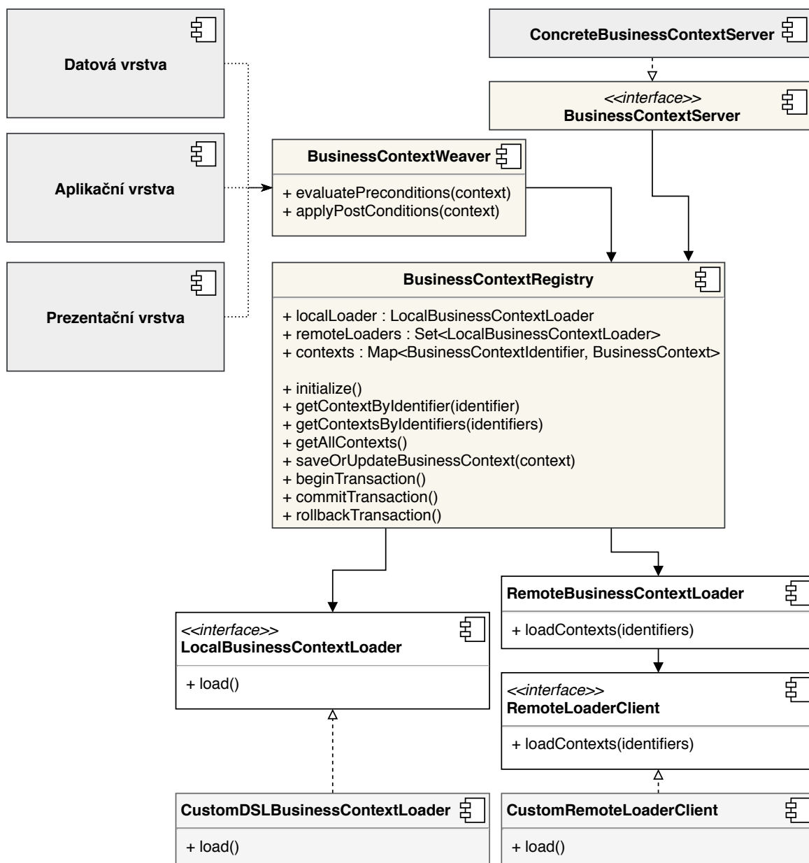
Obrázek 4.8: Architektura navrženého frameworku
