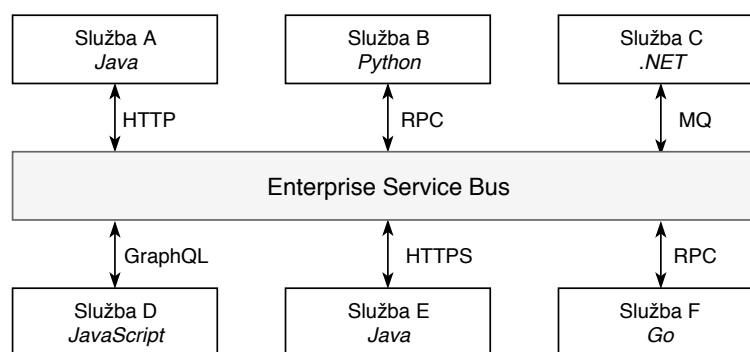
Obrázek 2.1: Komunikace služeb pomocí Enterprise Service Bus
