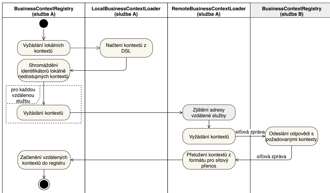
Obrázek 4.6: Proces inicializace byznysových kontextů
