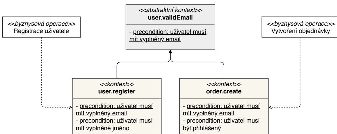
Obrázek 4.3: Znázornění abstraktního byznysového kontextu
