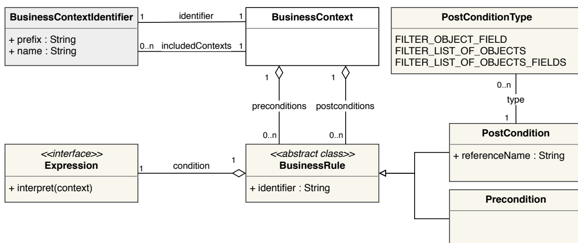
Obrázek 4.4: Metamodel byznysového kontextu
