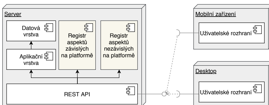
Obrázek 3.3: Architektura systému využívajícího ADDA
