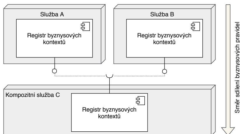
Obrázek 4.5: Postavení registrů byznysových kontextů vůči jednotlivým službám
