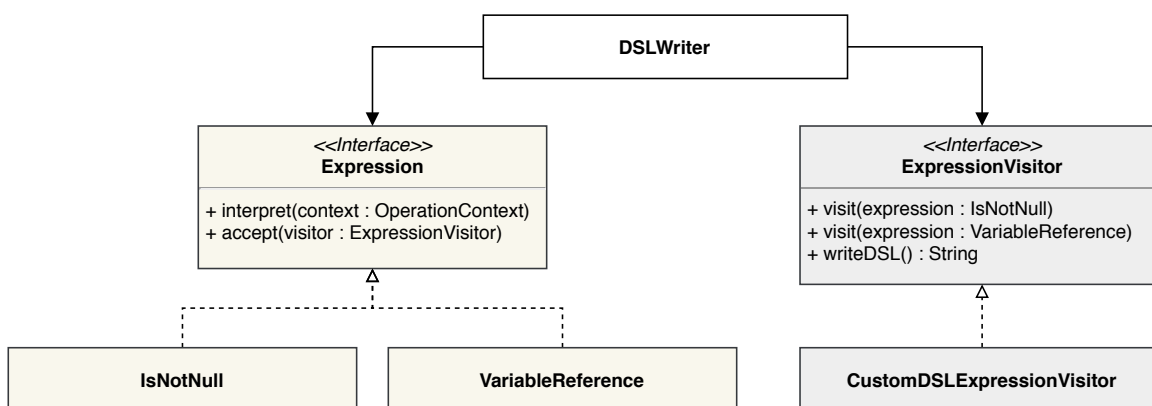
Obrázek 5.3: Využití vzoru Visitor pro převod logických výrazů do DSL
