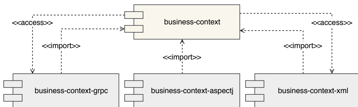
Obrázek 5.4: Moduly prototypu knihovny pro jazyk Java a jejich závislosti
