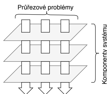
Obrázek 3.1: Průřezové problémy v informačních systémech
