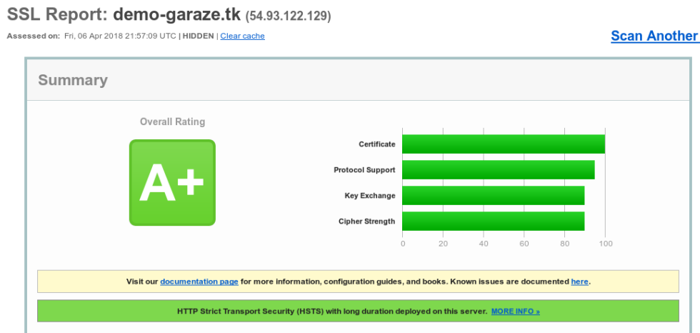
Obrázek 5.1: Výsledky testu HTTPS konfigurace poskytnutého společností Qualys.
