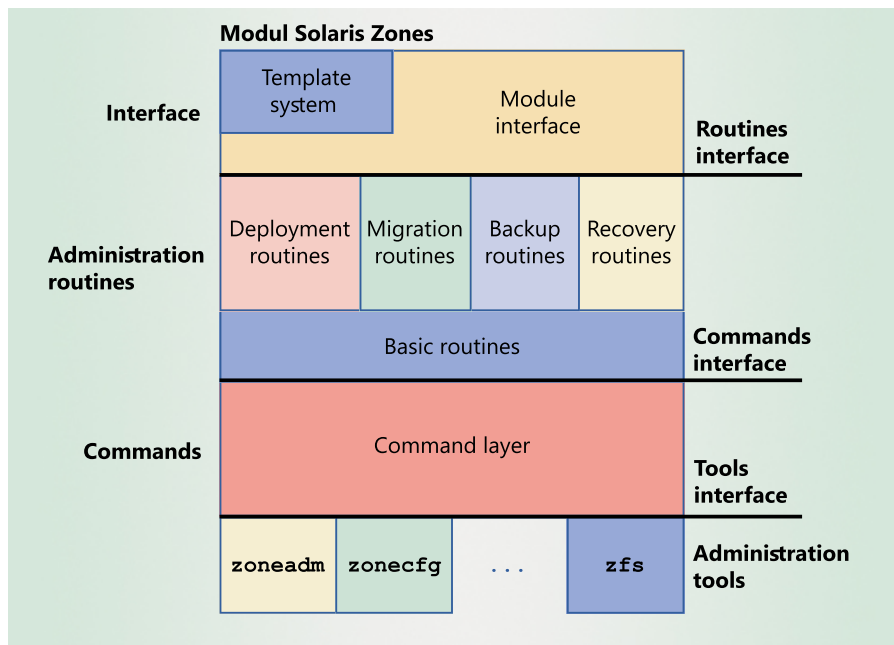
Obrázek 5.2: Architektura modulu Solaris Zones
