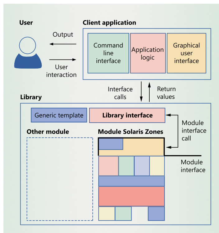
Obrázek 4.1: Architektura funkčních bloku aplikace
