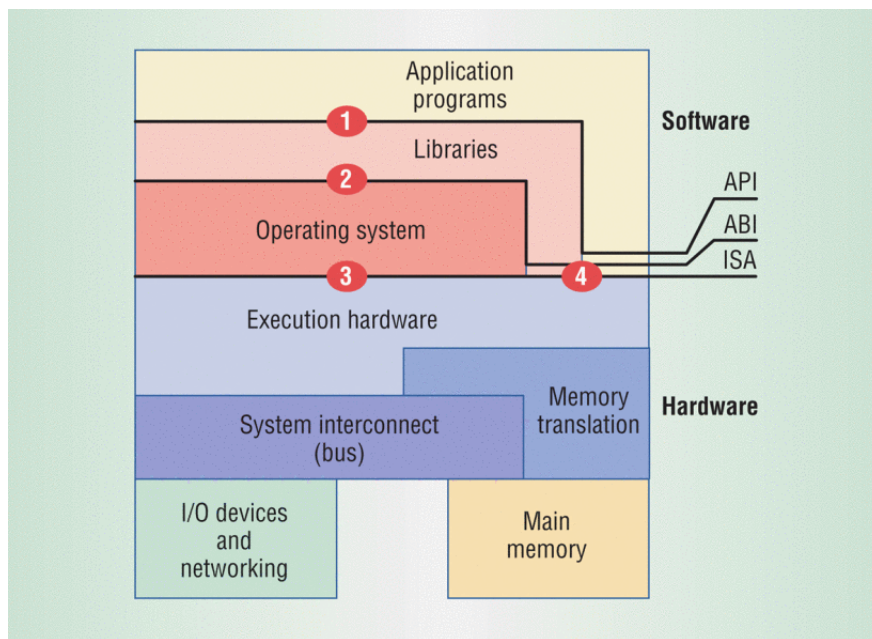
Obrázek 1.1: Architektura počítačového systému [3]
