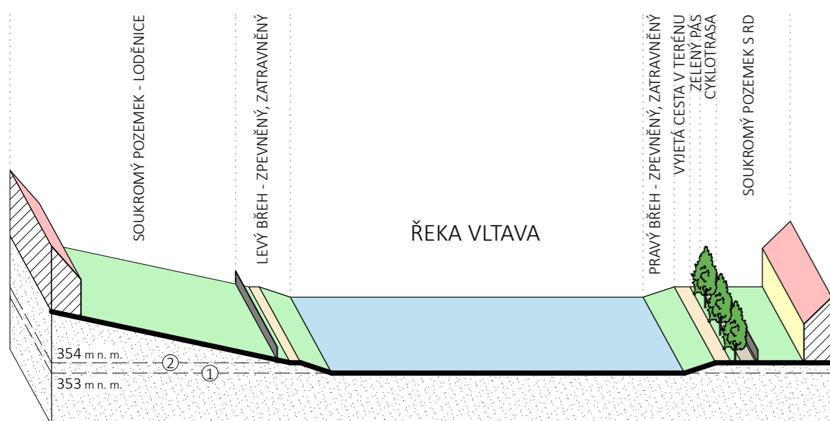
SCHÉMA ŘEZU C-C'
