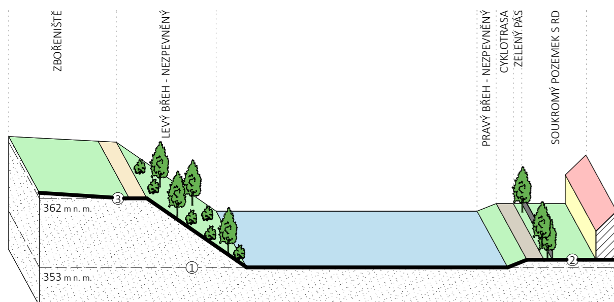
SCHÉMA ŘEZU B-B'
