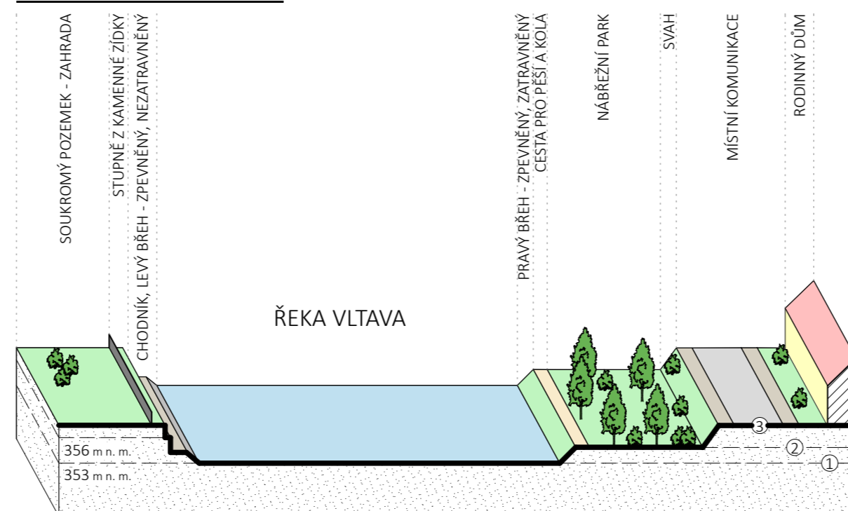
SCHÉMA ŘEZU D-D'
