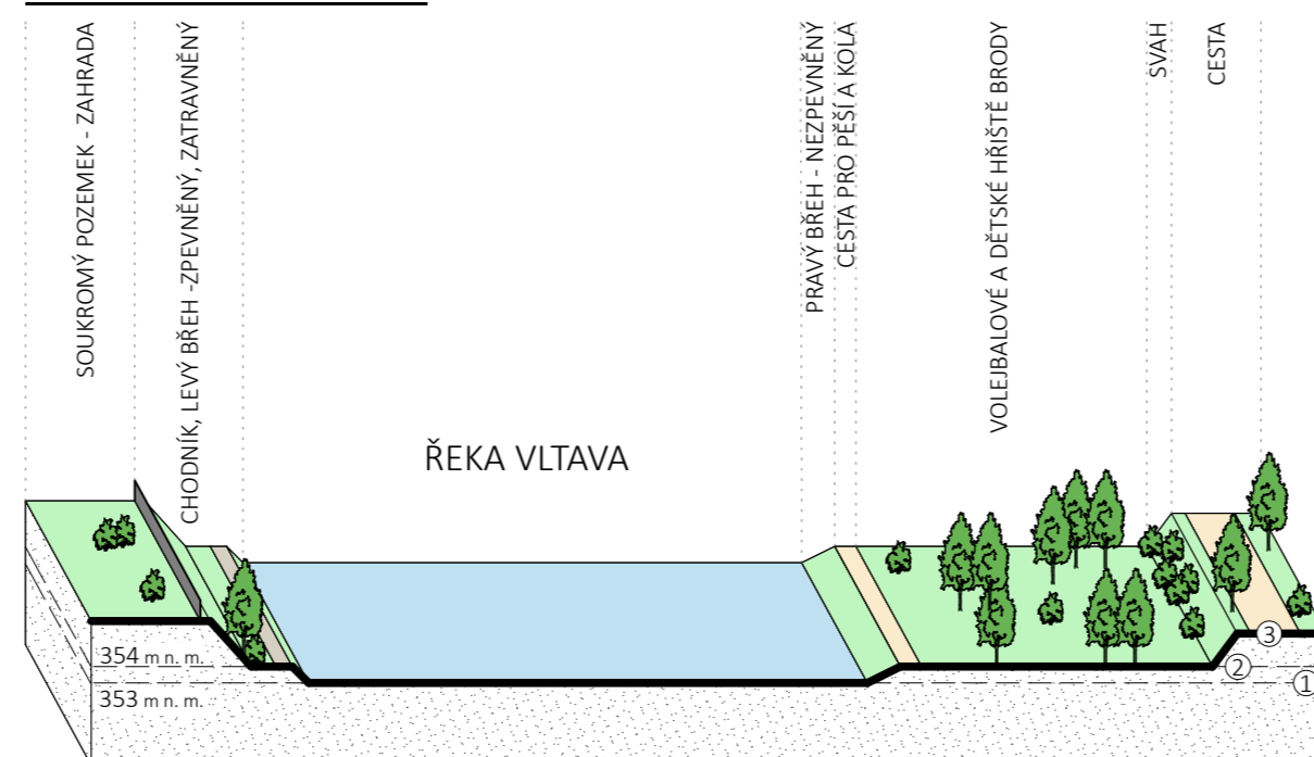
SCHÉMA ŘEZU E-E'
