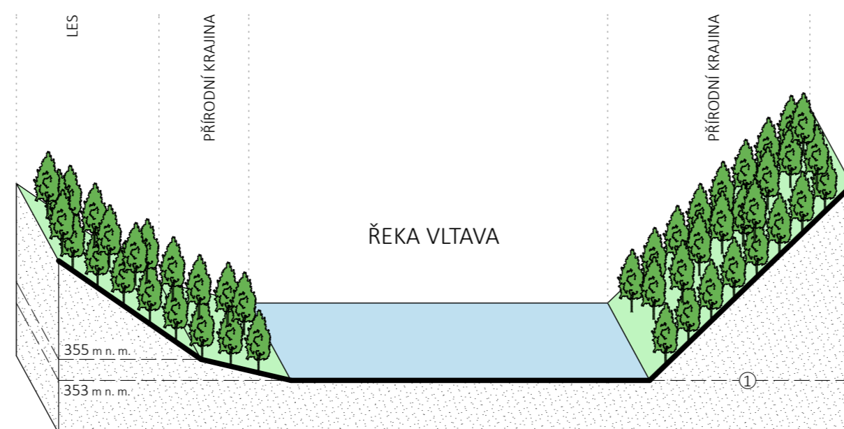
SCHÉMA ŘEZU F-F'
