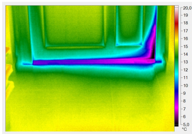
Ilustrace 8: Tepelný únik - spodní část vstupních dveří
