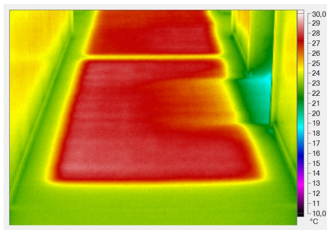
Ilustrace 9: Únik tepla pode dveřmi mezi chodbou a předsíní
