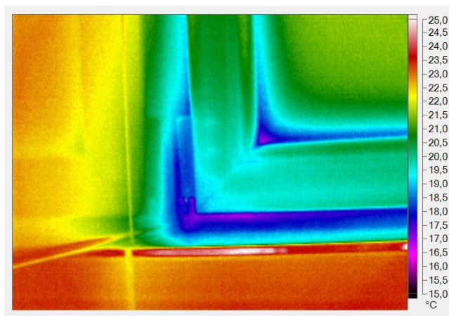
Ilustrace 6: Tepelný únik - pant okna v koupelně
