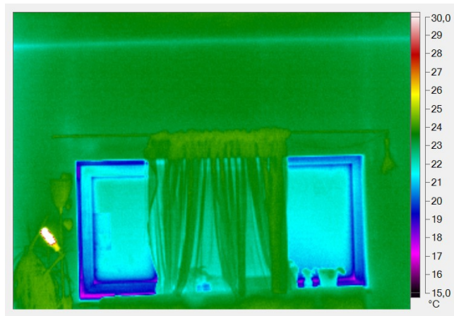
Ilustrace 11: Termogram okna v obývacím pokoji
