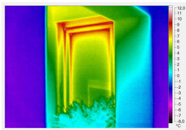
Ilustrace 2: Únik tepla - okno koupelna
