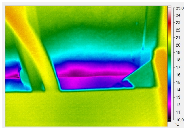
Ilustrace 4: Únik tepla v místě prostupu vodovodu a kanalizace do objektu pod kuchyňským dřezem
