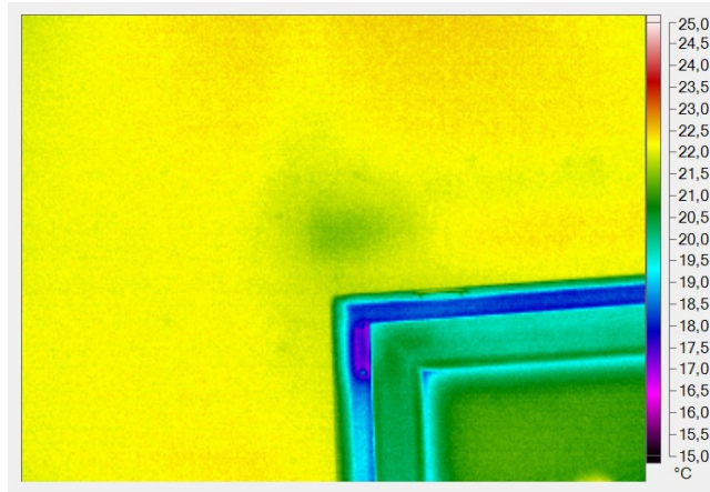
Ilustrace 7: Tepelný únik - pant okna; ochlazované místo nad rohem otvoru - pravděpodobně prostupu pro ovládaní žaluzií
