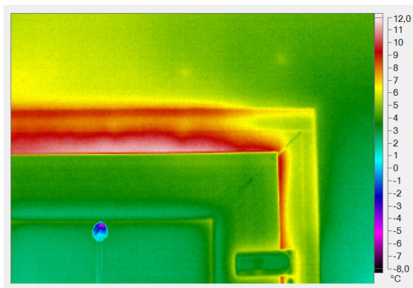
Ilustrace 1: Únik tepla mezi křídlem a rámem vstupních dveří
