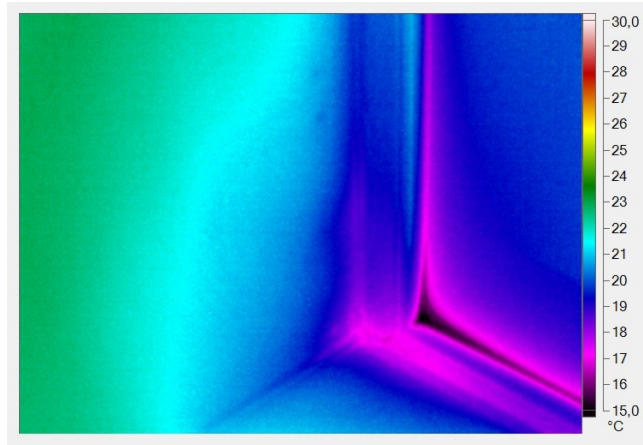
Ilustrace 10: Tepelný únik v místě usazení skla do rámu
