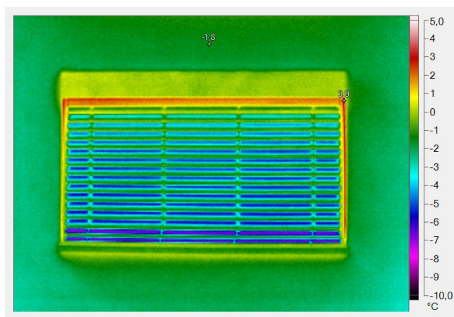
Ilustrace 3: Termogram okna
