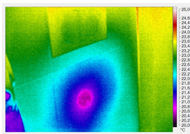
Ilustrace 5: Ochlazované místo - modul závěsného WC v koupelně
