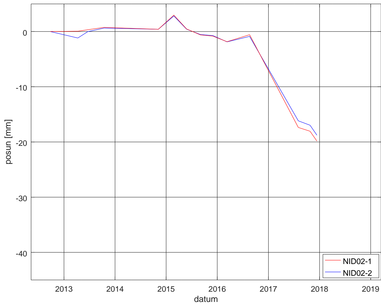
Vyvoj posunu na profilu NID02
