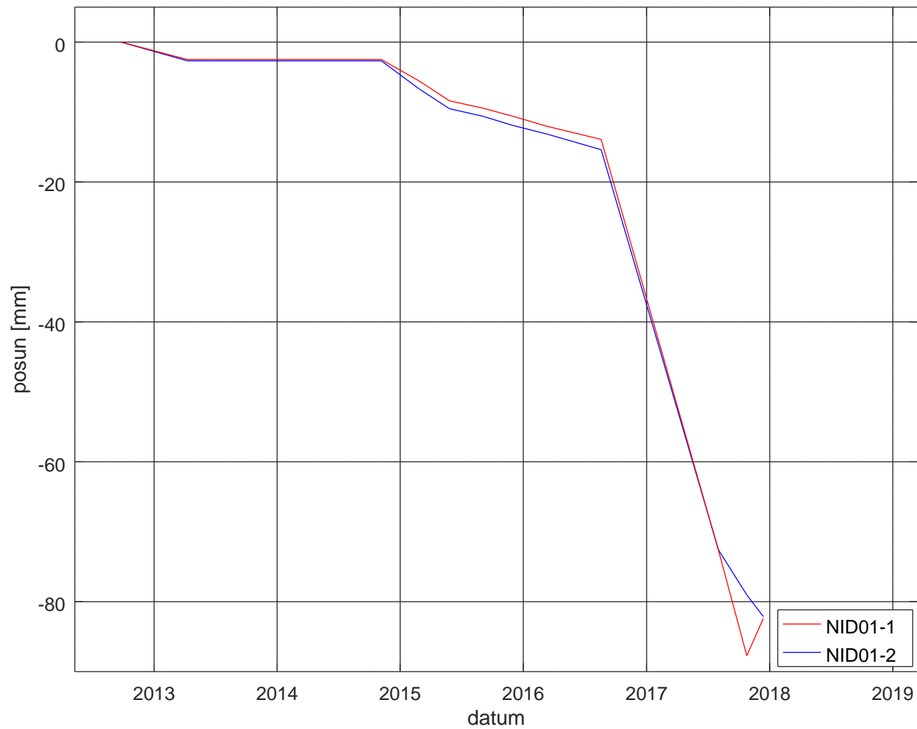
Vyvoj posunu na profilu NID01
