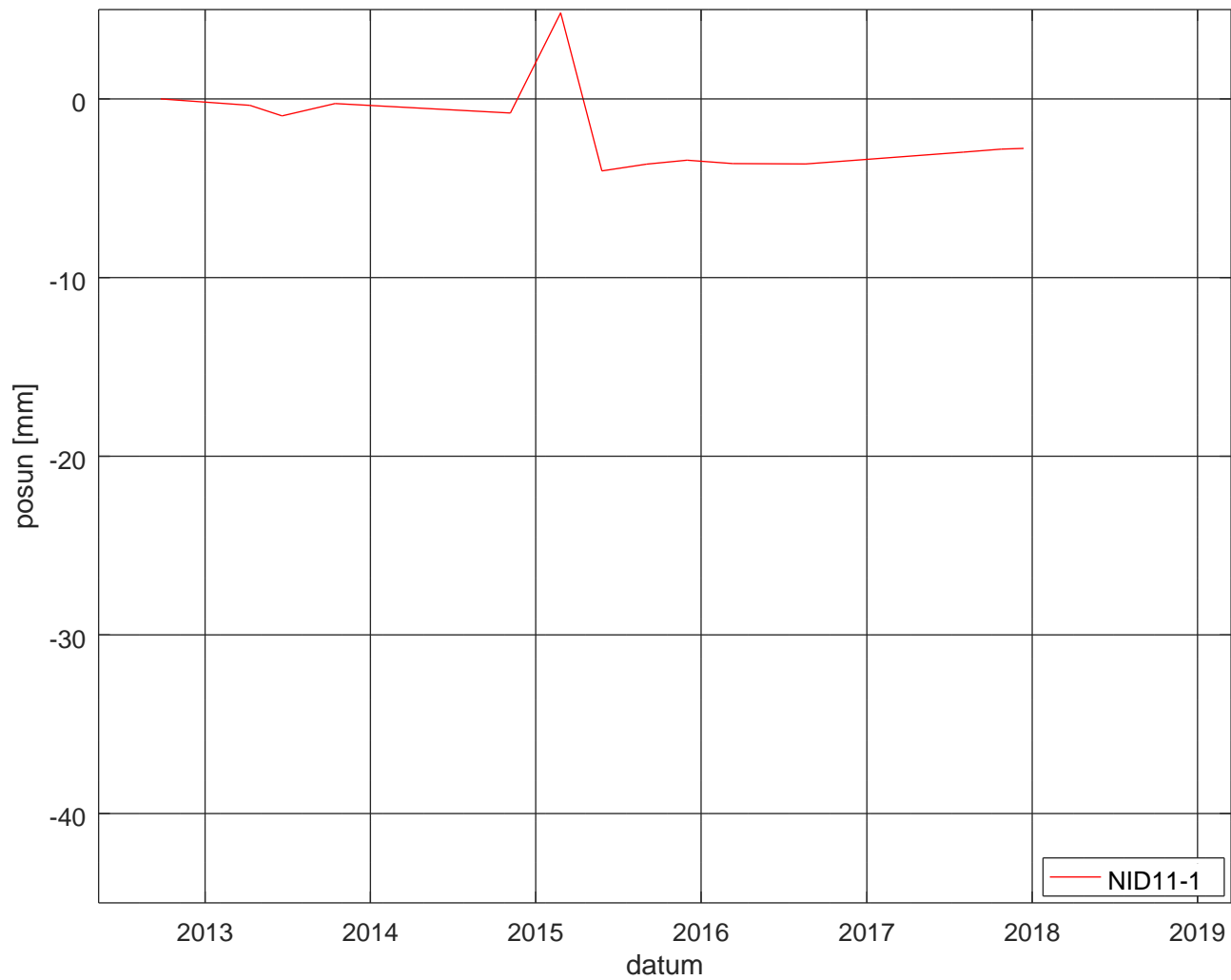
Vyvoj posunu na profilu NID11
