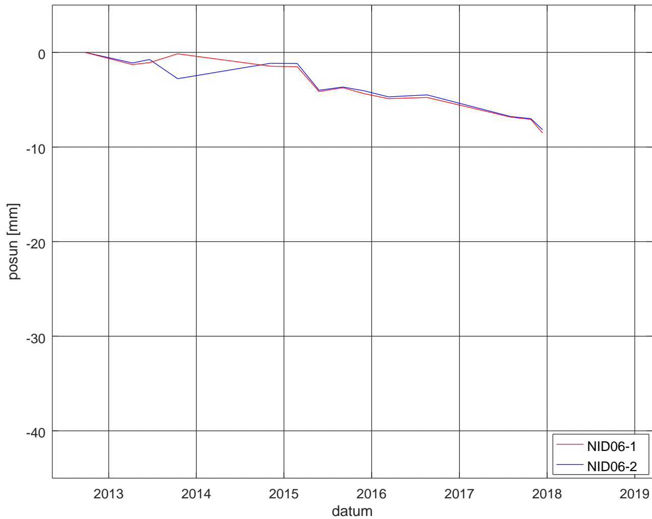
Vyvoj posunu na profilu NID06
