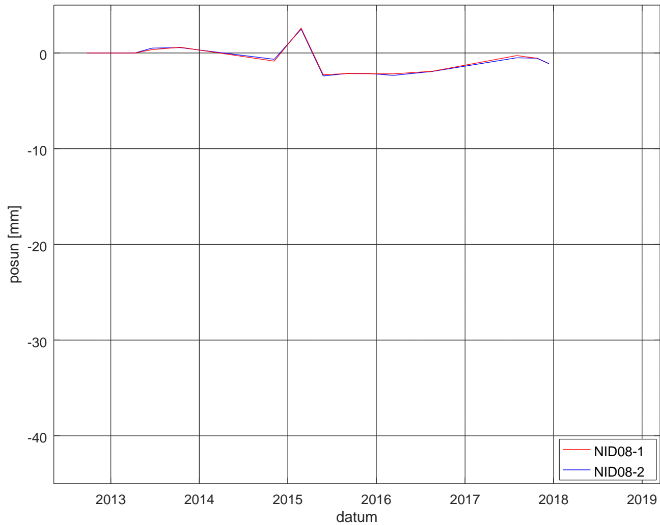
Vyvoj posunu na profilu NID08
