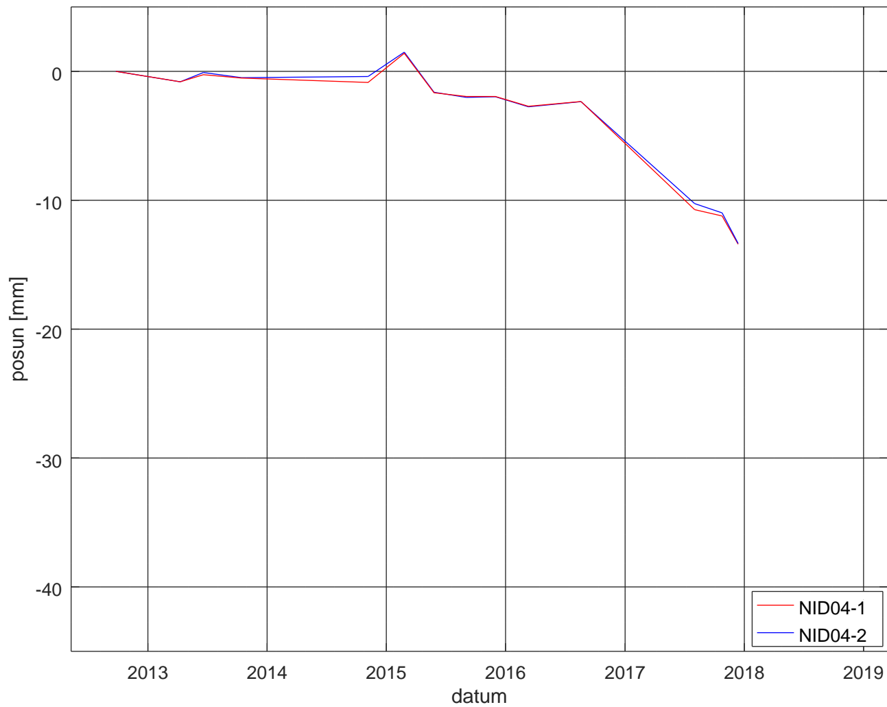
Vyvoj posunu na profilu NID04
