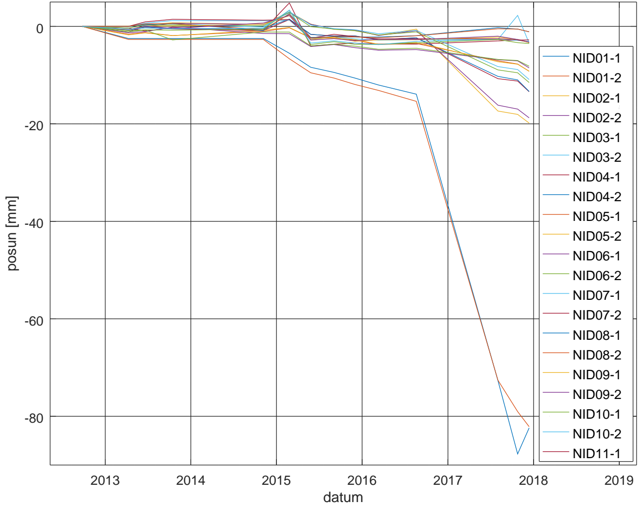
Vyvoj posunu vseh bodu
