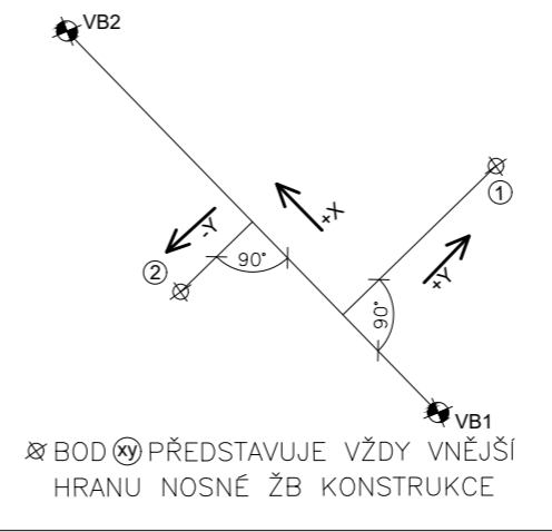
TABULKA PRO VYTYČENÍ OBJEKTU + SCHÉMA VYTYČOVÁNÍ
